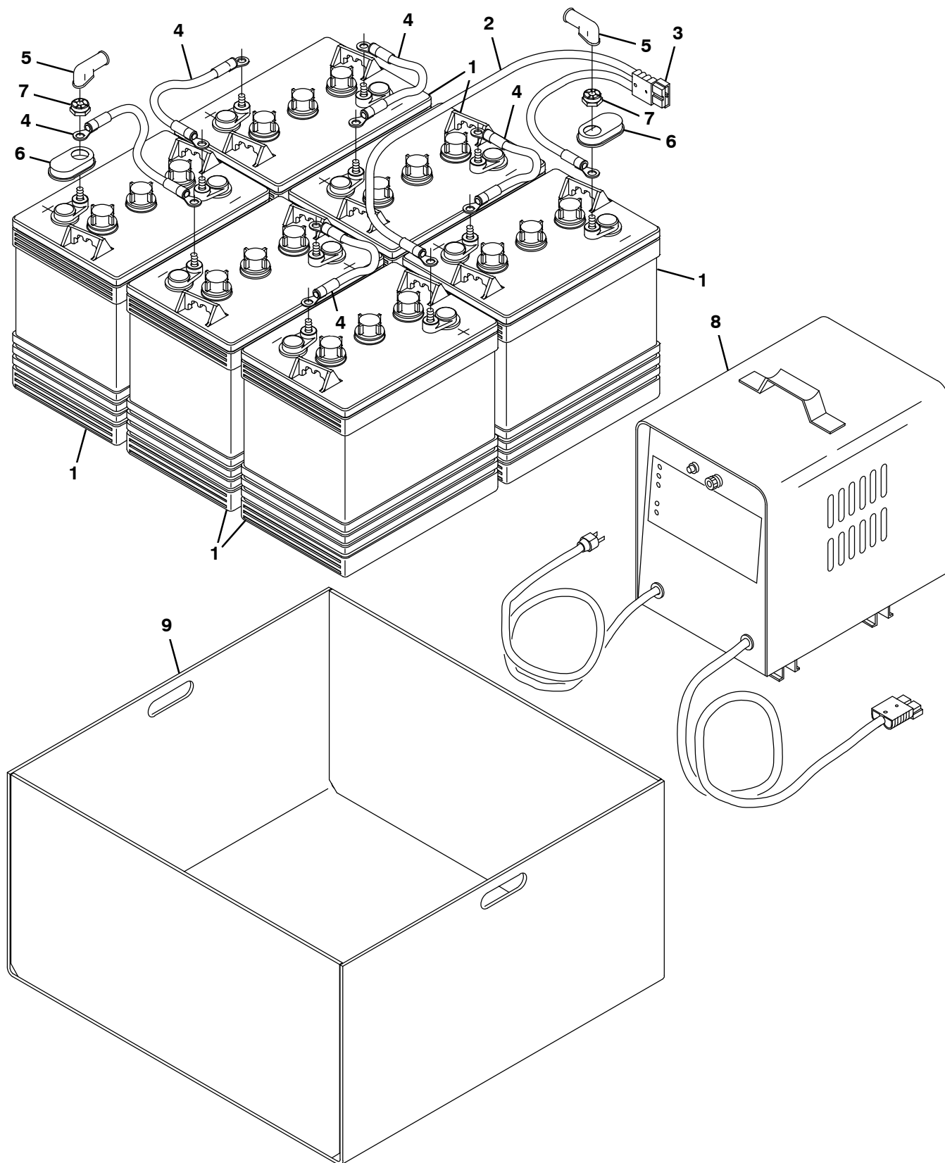
Fig. 14 – Rollout Battery and Charger Group, 220AH (0001–4000) — Ausrollbatterie- und Ladegerät-Einheit, 220AH (0001–4000) — Groupe batterie amovible et chargeur 220AH (0001–4000)
