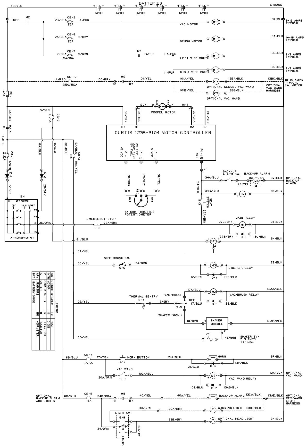
Fig. 31 – Electrical Schematic (6100 0256– ) — Elektroschema (6100 0256– ) — Schéma des connexions électriques (6100 0256– )
