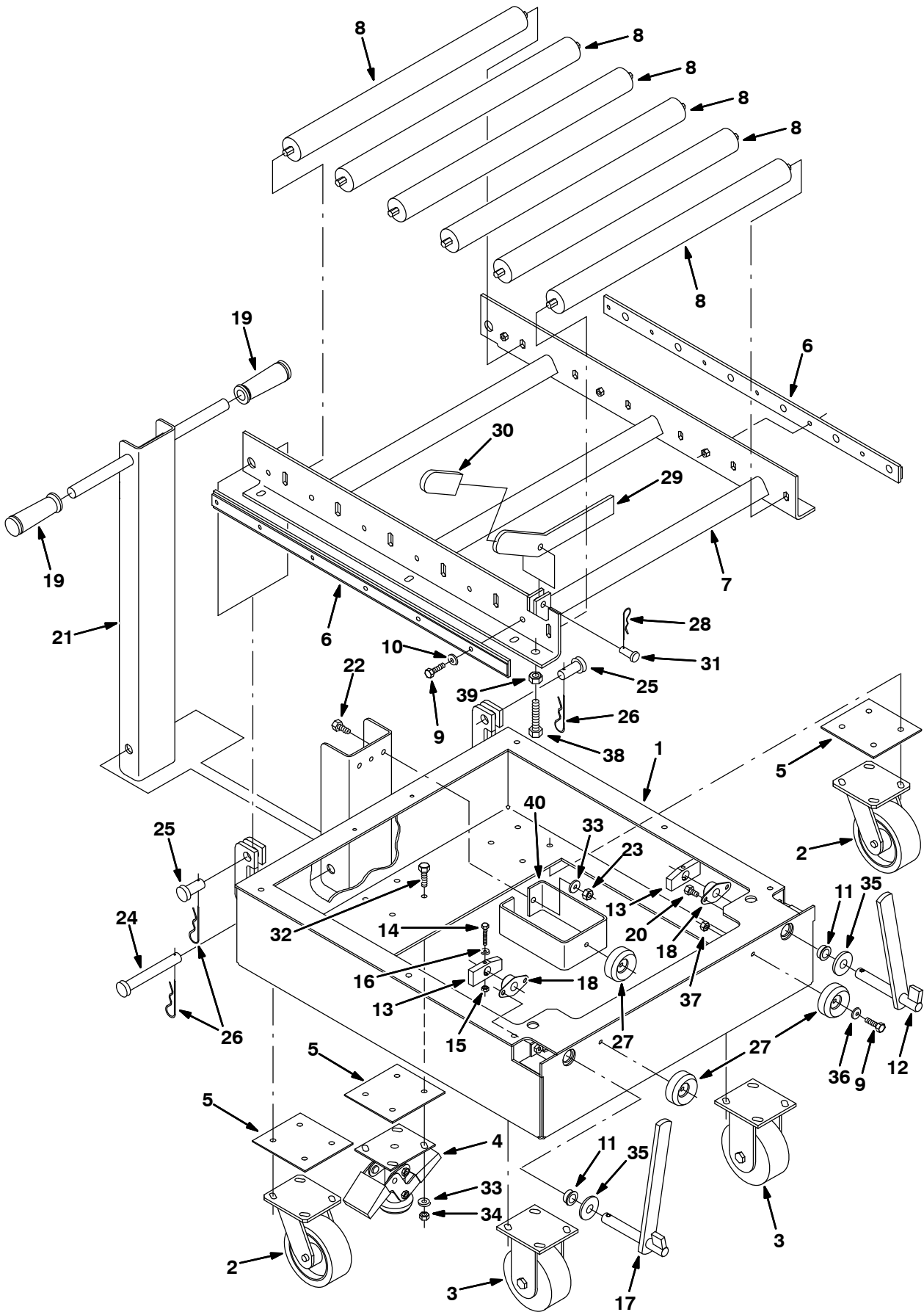
Fig. 10 – Rollout Battery Cart Kit (0001–4000) — Transporteinheit für Ausroll-Batterien (0001–4000) — Lot meuble roulant pour batteries sur roulettes (0001–4000)
