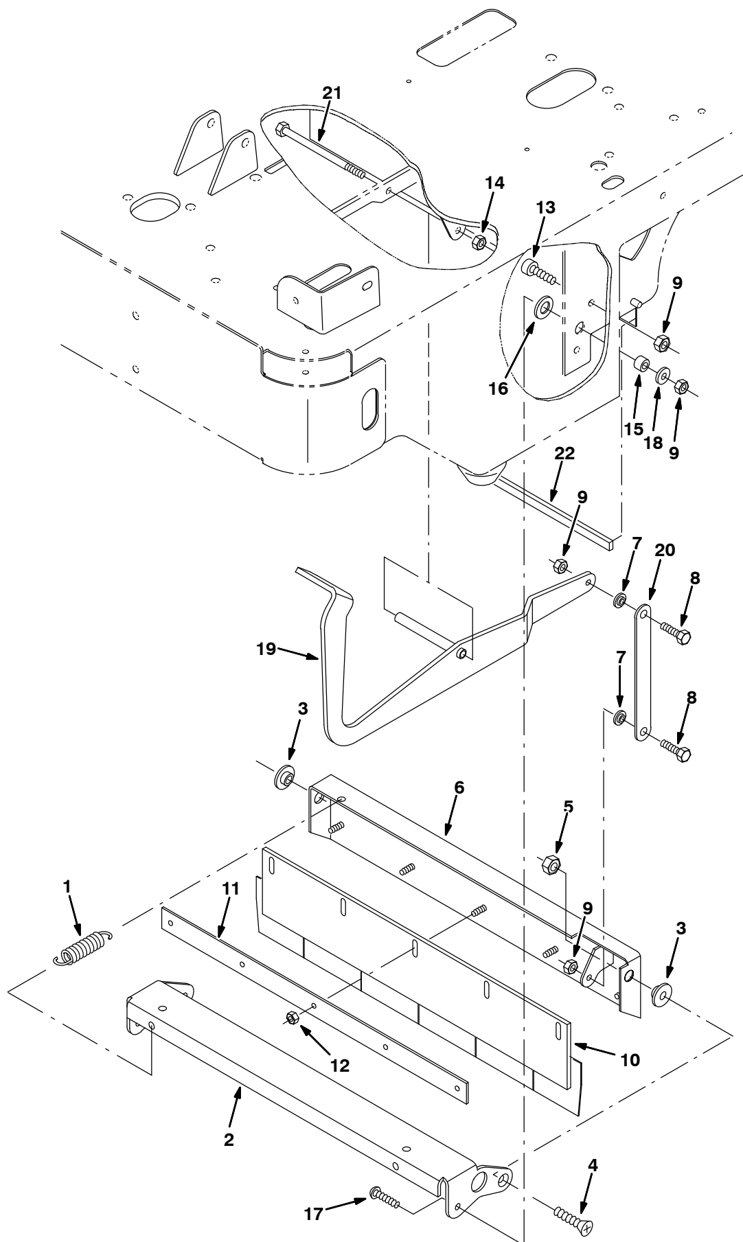
Fig. 20 – Main Brush Front Flap Group — Hauptbürsten-Vorderklappen-Gruppe — Groupe jupes de la brosse principale
