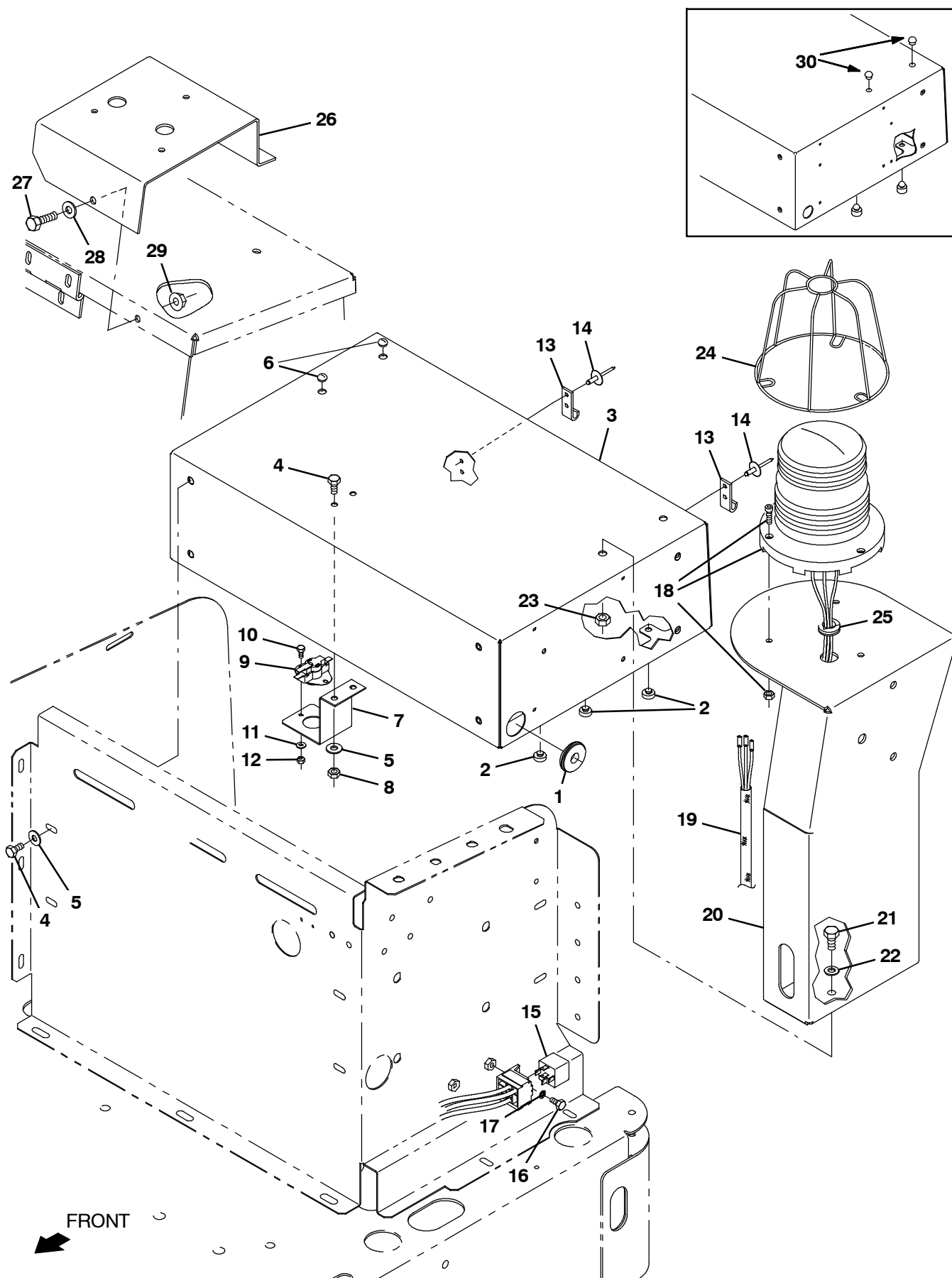
Fig. 26 - Vacuum Fan Box Group — Saugventilator-Verpackungs-Gruppe — Groupe châssis de l'extracteur
