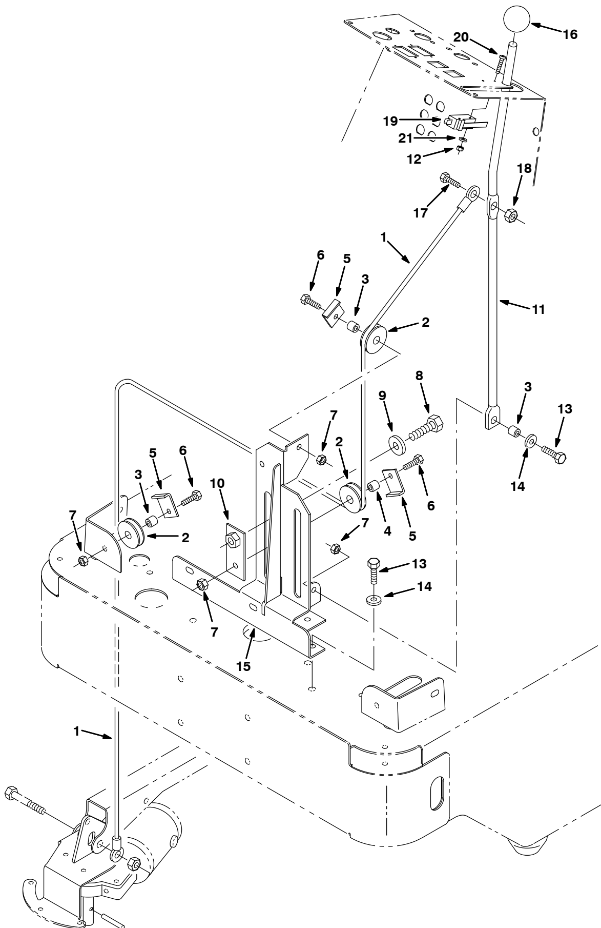
Fig. 23 – Side Brush Lift Group — Seitenbürsten-Hebe-Gruppe — Groupe levage de la brosse latérale
