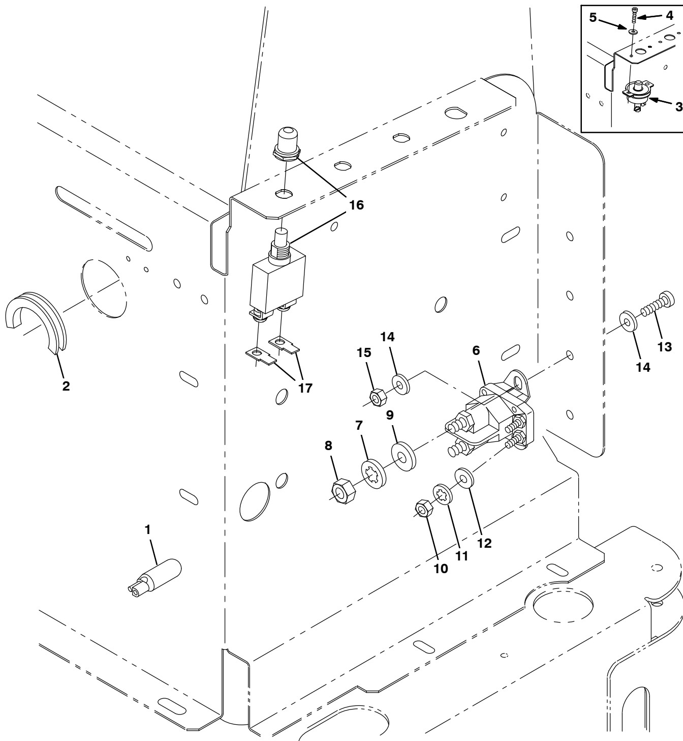
Fig. 6 – Vacuum Wand Electrical Group, Dual Fan — Saugstab-Elektrik-Gruppe, Doppelentilator — Système électrique du manche d'aspiration, double extracteur
