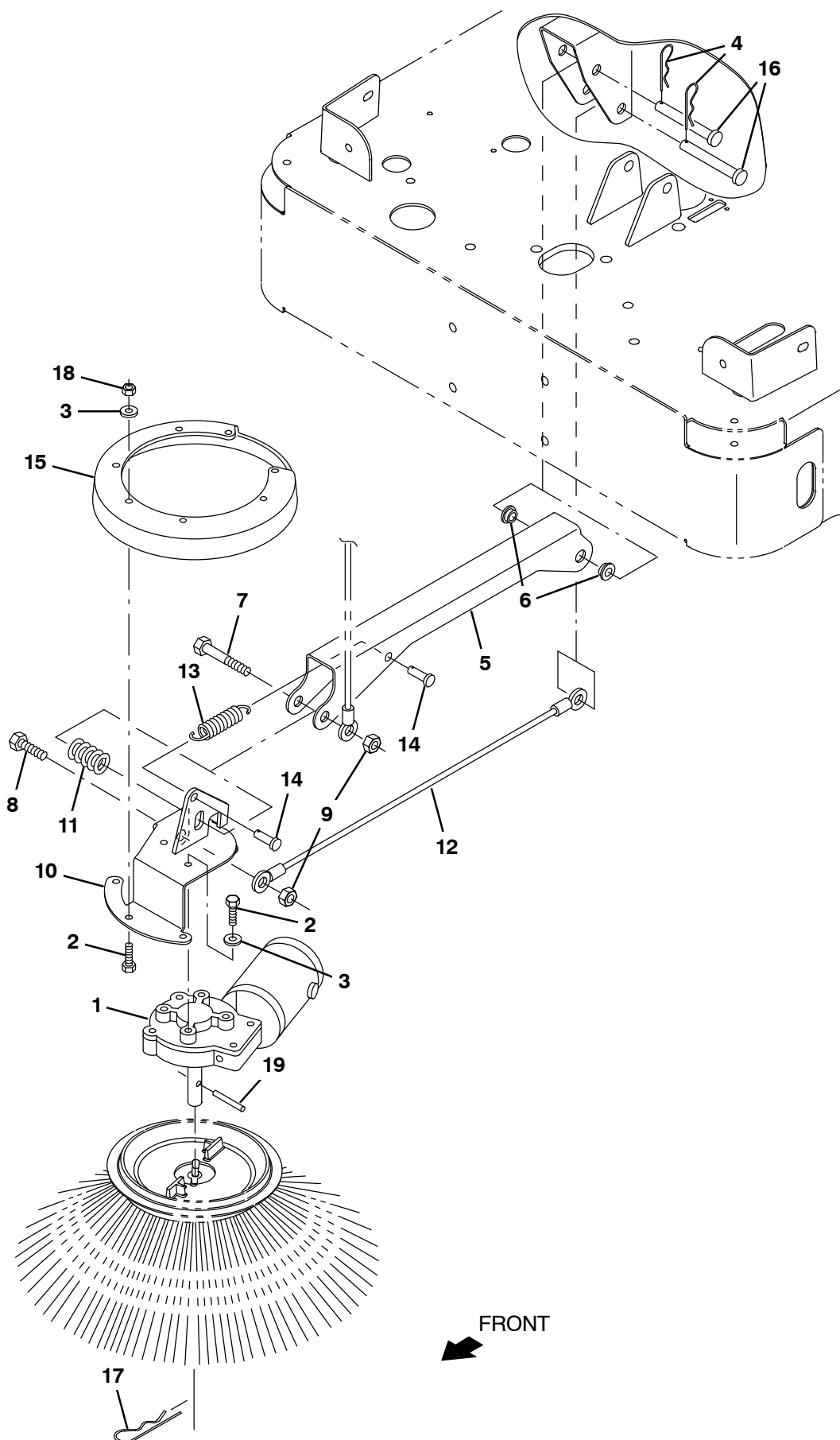
Fig. 24 – Side Brush Motor Group — Seitenbürsten-Motorgruppe — Groupe moteur de la brosse latérale
