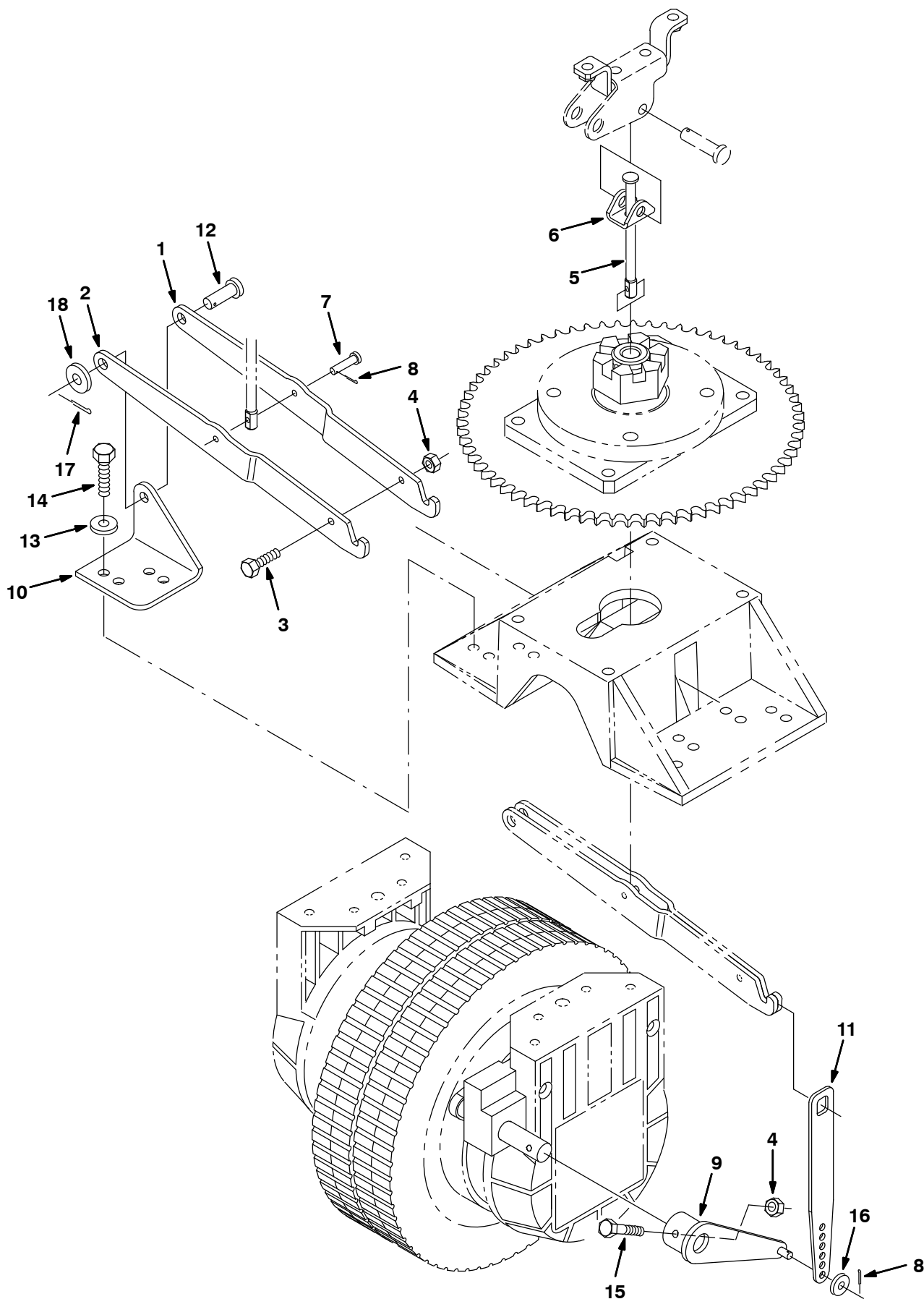
Fig. 14 – Front Brake Linkage Group (6100530 823- ) — Vorderbremsen-Gestänge-Gruppe (6100530 823- ) — Assemblage timonerie des freins avant (6100530 823- )
