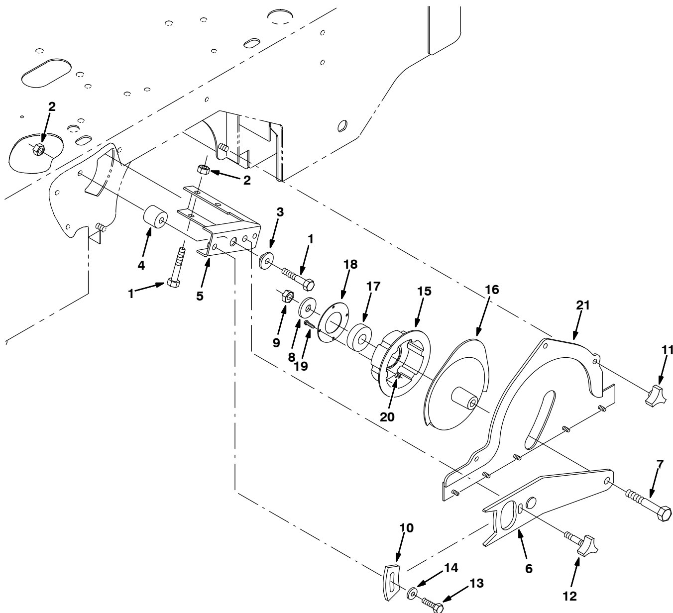
Fig. 21 – Main Brush Idler Group — Hauptbürsten-Leerlaufnaben-Gruppe — Groupe pignon de renvoi de la brosse principale
