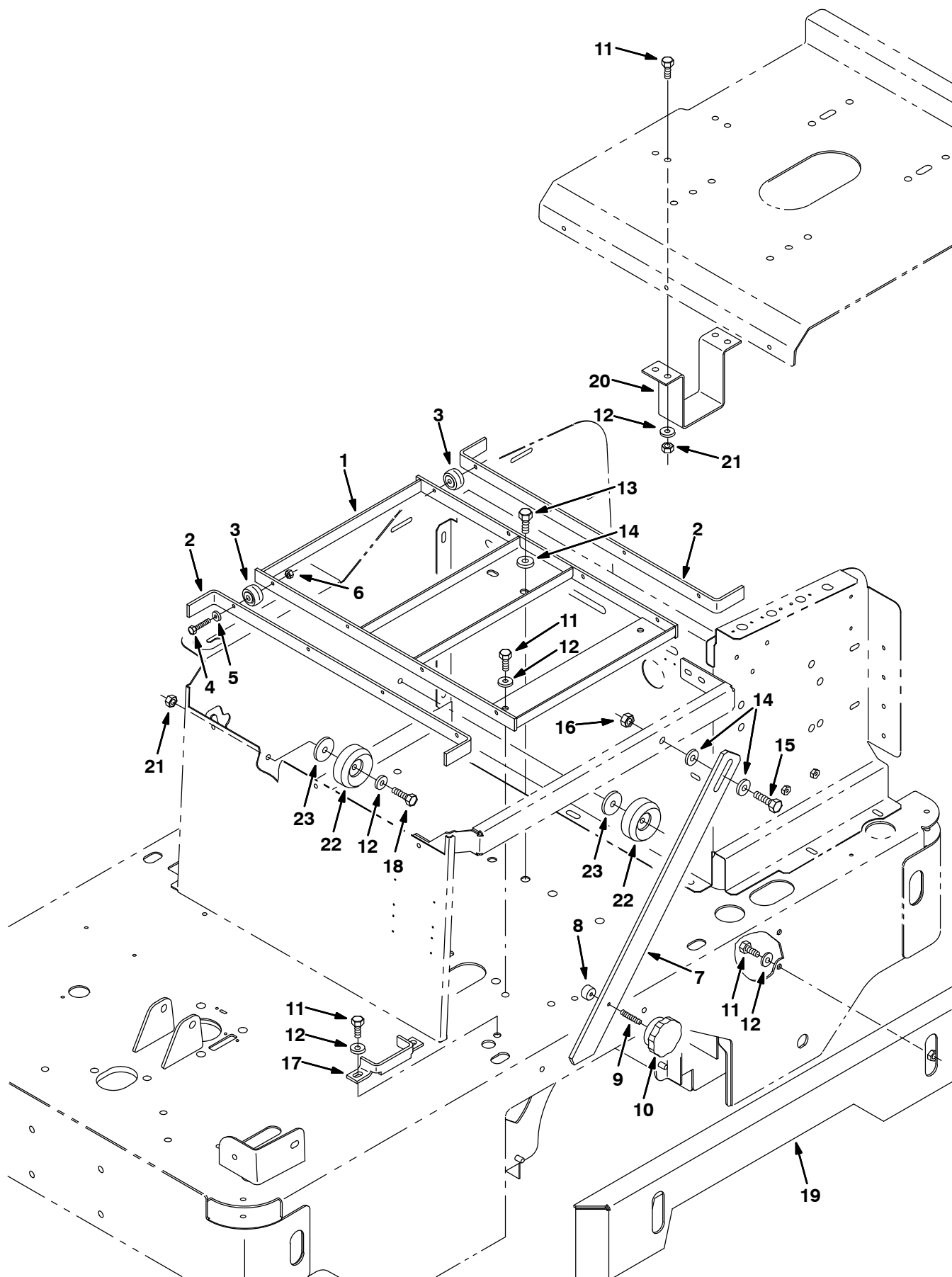
Fig. 9 – Rollout Battery Case Kit (0001–4000) — Gehäuse der Ausroll-Batterie (0001–4000) — Groupe logement des batteries sur roulettes (0001–4000)
