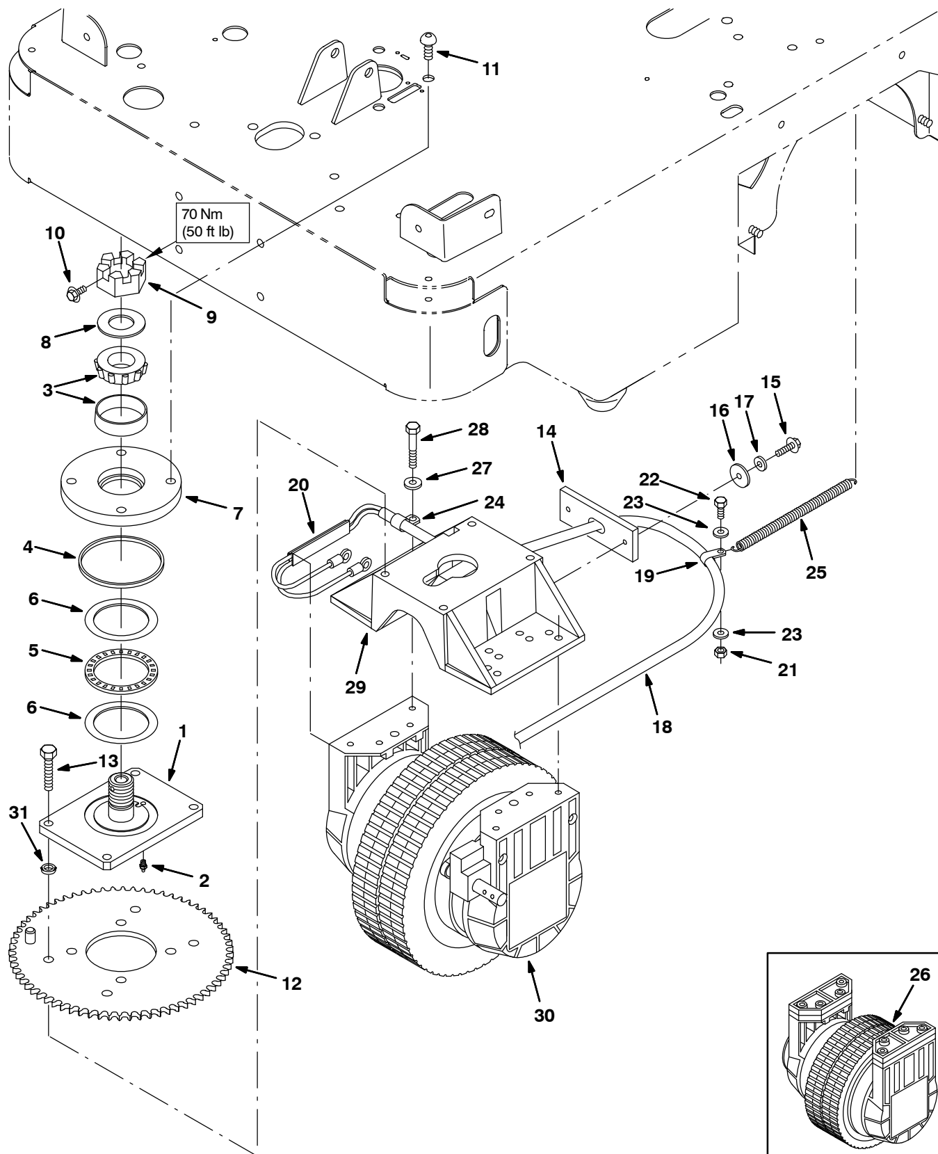
Fig. 11 – Front Drive Wheel Group (6100530 729– ) — Vorderantrieb-Rad-Gruppe (6100530 729– ) — Groupe roues motrices avant (6100530 729– )
