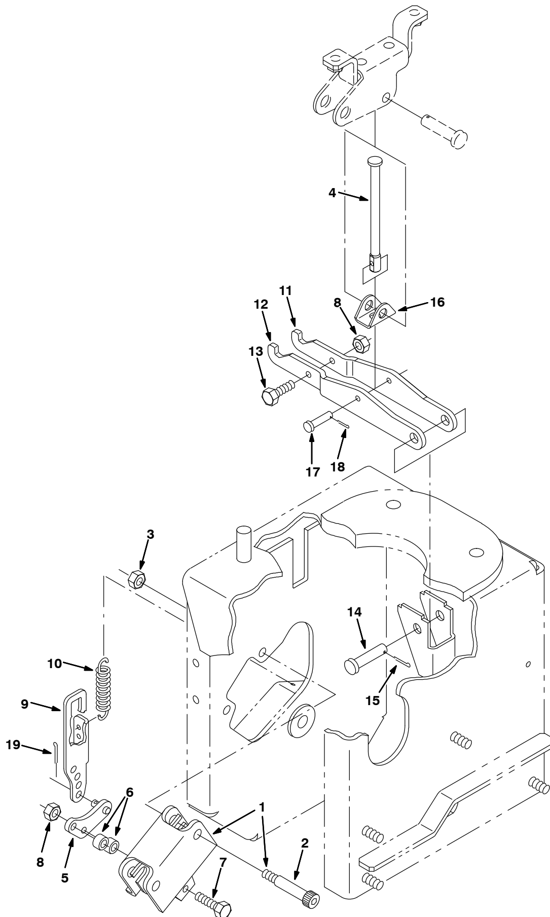
Fig. 12 – Front Brake Linkage Group (6100530 001-728) — Vorderbremsen-Gestänge-Gruppe (6100530 001-728) — Assemblage timonerie des freins avant (6100530 001-728)
