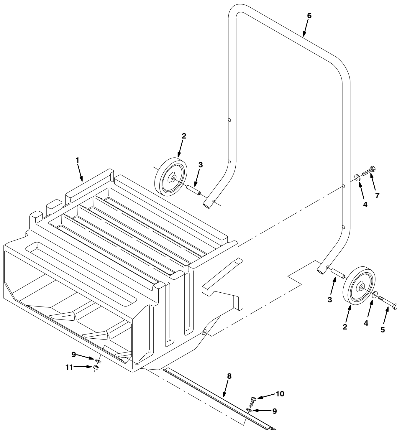
Fig. 27 – Hopper Group — Kehrlichtbehälter-Gruppe — Groupe trémie
