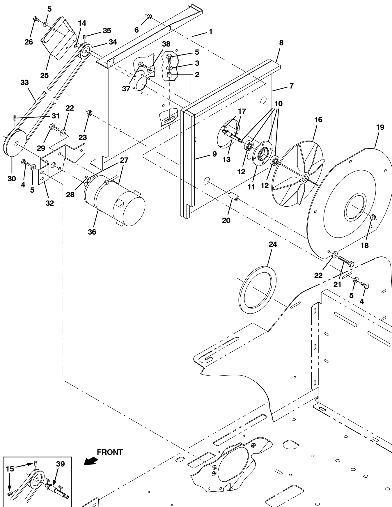
Fig. 25 – Vacuum Fan Group — Vakuumbelüftung-Gruppe — Groupe extracteur
