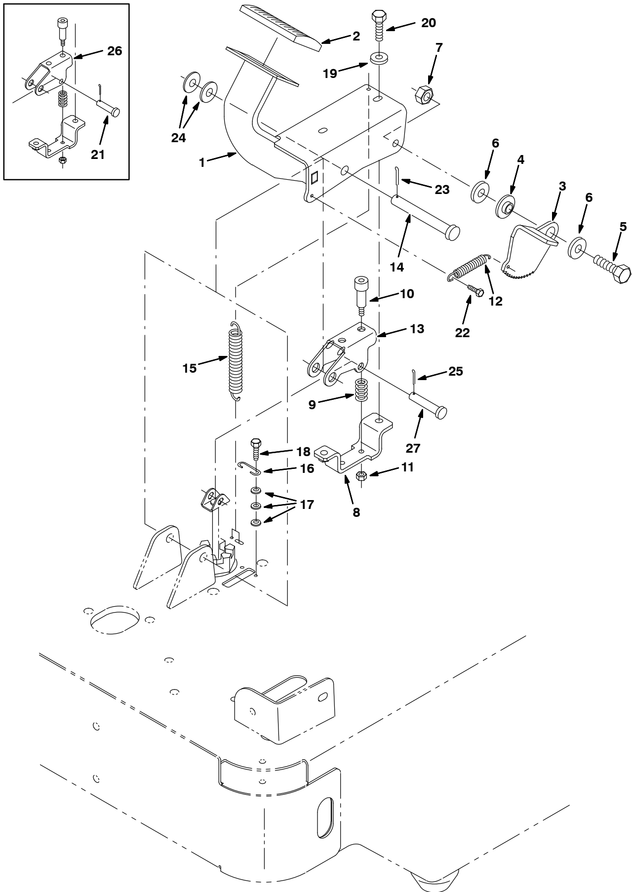
Fig. 18 – Brake Pedal Group — Bremspedal-Gruppe — Groupe pédale de frein
