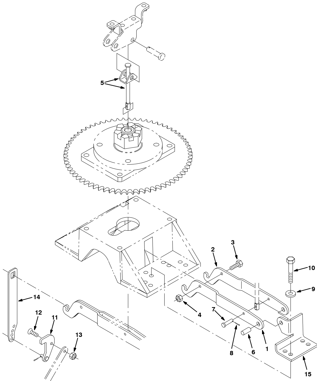
Fig. 13 – Front Brake Linkage Group (6100530 729–822) — Vorderbremsen-Gestänge-Gruppe (6100530 729–822) — Assemblage timonerie des freins avant (6100530 729–822)
