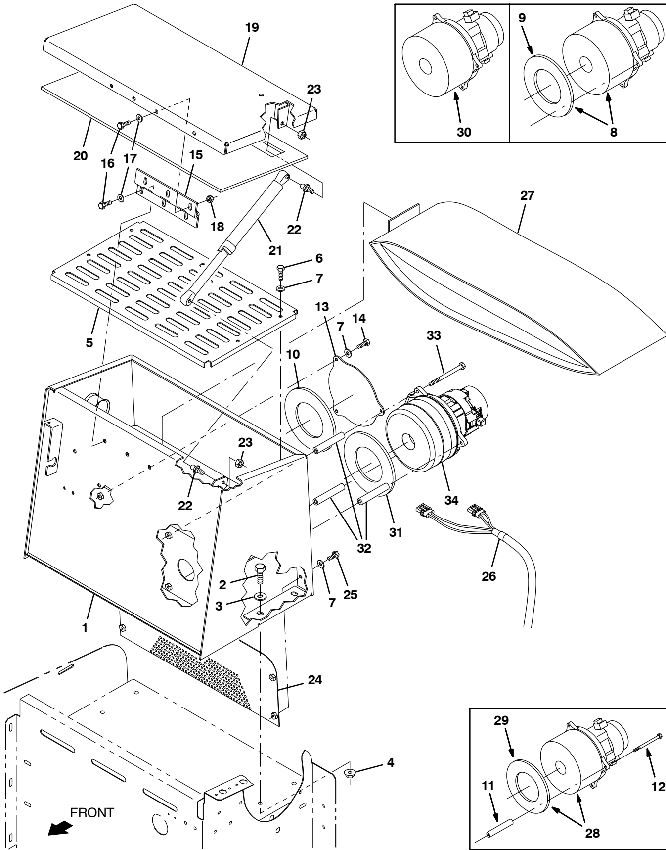
Fig. 3 – Vacuum Wand Box Group, Single Fan — Saugstab-Verpackungs-Gruppe, Einzelventilator — Groupe châssis du manche d’aspiration, extracteur simple
