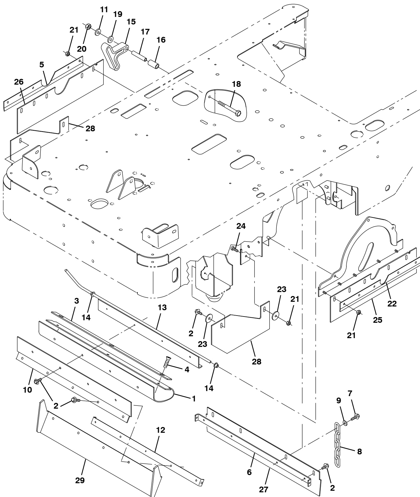
Fig. 19 – Main Brush Skirts Group — Hauptbürsten-Schürzen-Gruppe — Groupe jupes de la brosse principale
