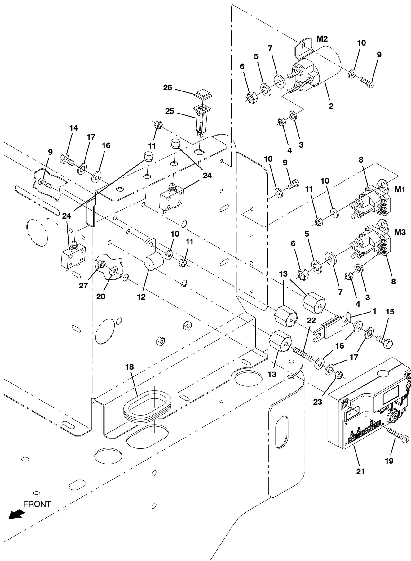
Fig. 8 – Electrical Panel Group (3012- ) — Elektronik-Schaltfeld-Gruppe (3012- ) — Assemblage tableau électronique (3012- )
