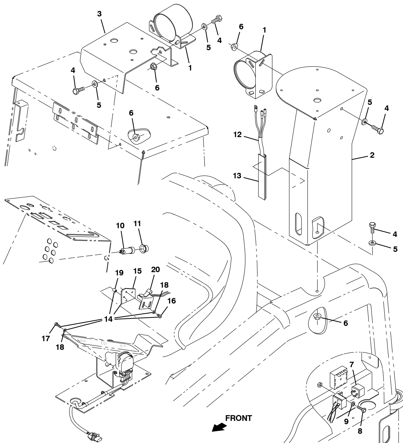
Fig. 12 – Backup Alarm Kit (6100 0001–0906) — Rückfahr-Alarm-Satz (6100 0001–0906) — Jeu de pièces alarme de sécurité (6100 0001–0906)
