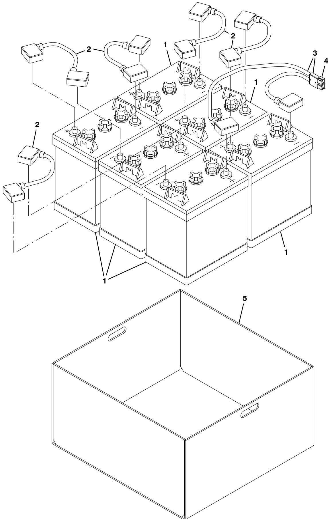
Fig. 15 – Rollout Battery Group, 185AH (0001–4000) — Ausrollbatterie Einheit, 185AH (0001–4000) — Groupe batterie 185AH (0001–4000)
