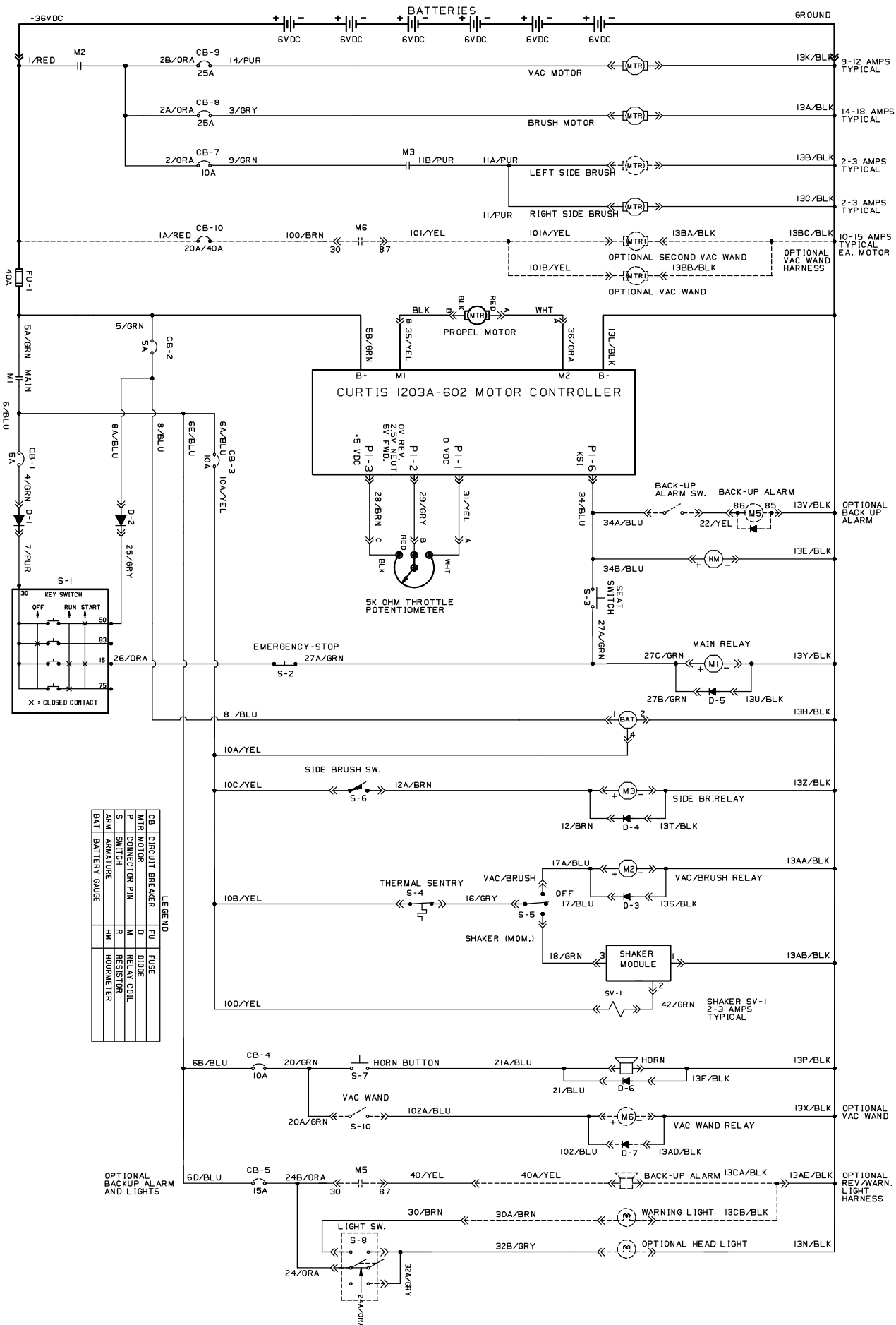
Fig. 30 – Electrical Schematic (6100 0001–0255) — Elektroschaltbild (6100 0001–0255) — Schéma Électrique (6100 0001–0255)
