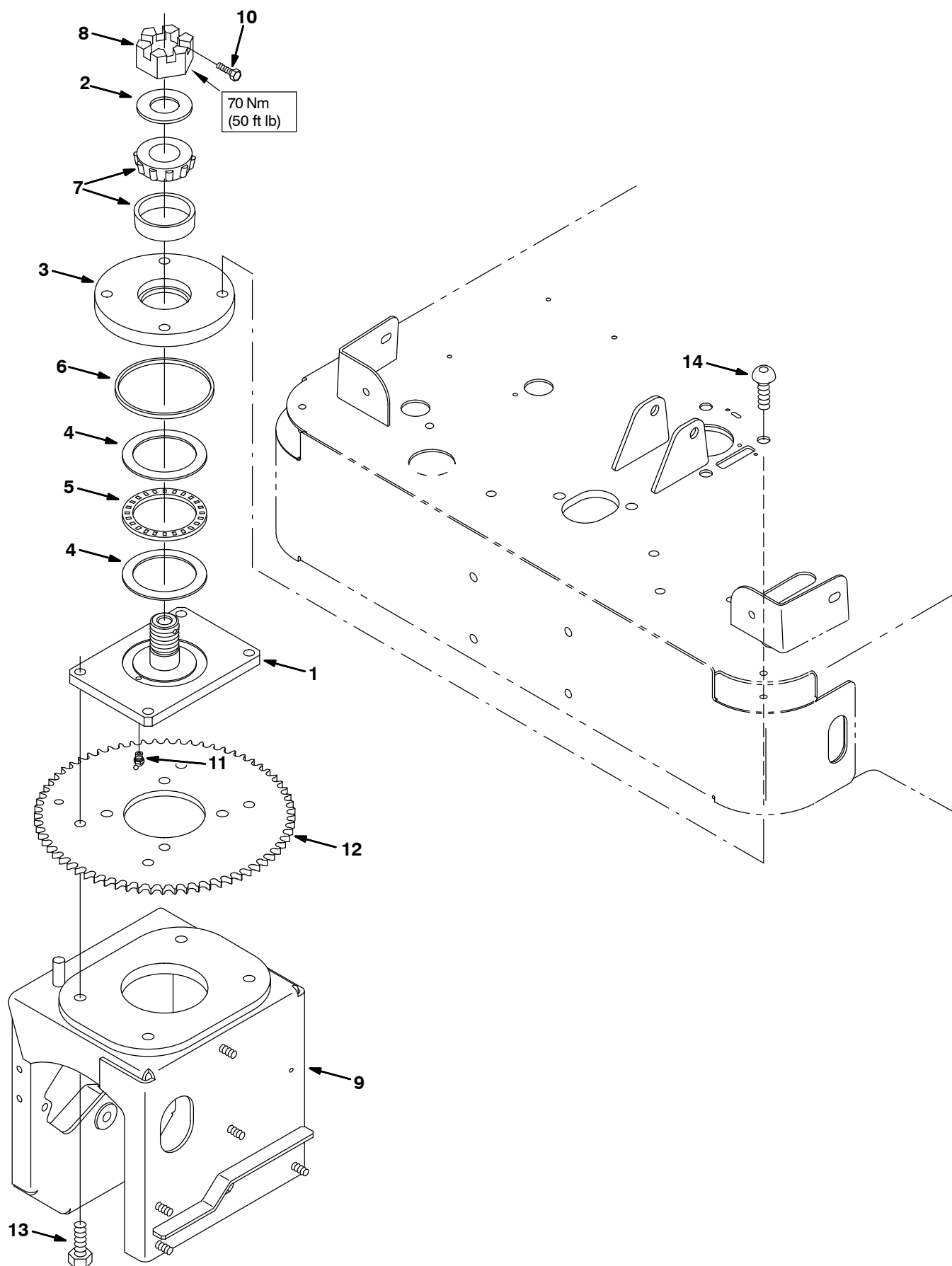
Fig. 9 – Front Wheel Pivot Group (6100530 001–728) — Vorderradgelenk-Gruppe (6100530 001–728) — Groupe rotule roue avant (6100530 001–728)
