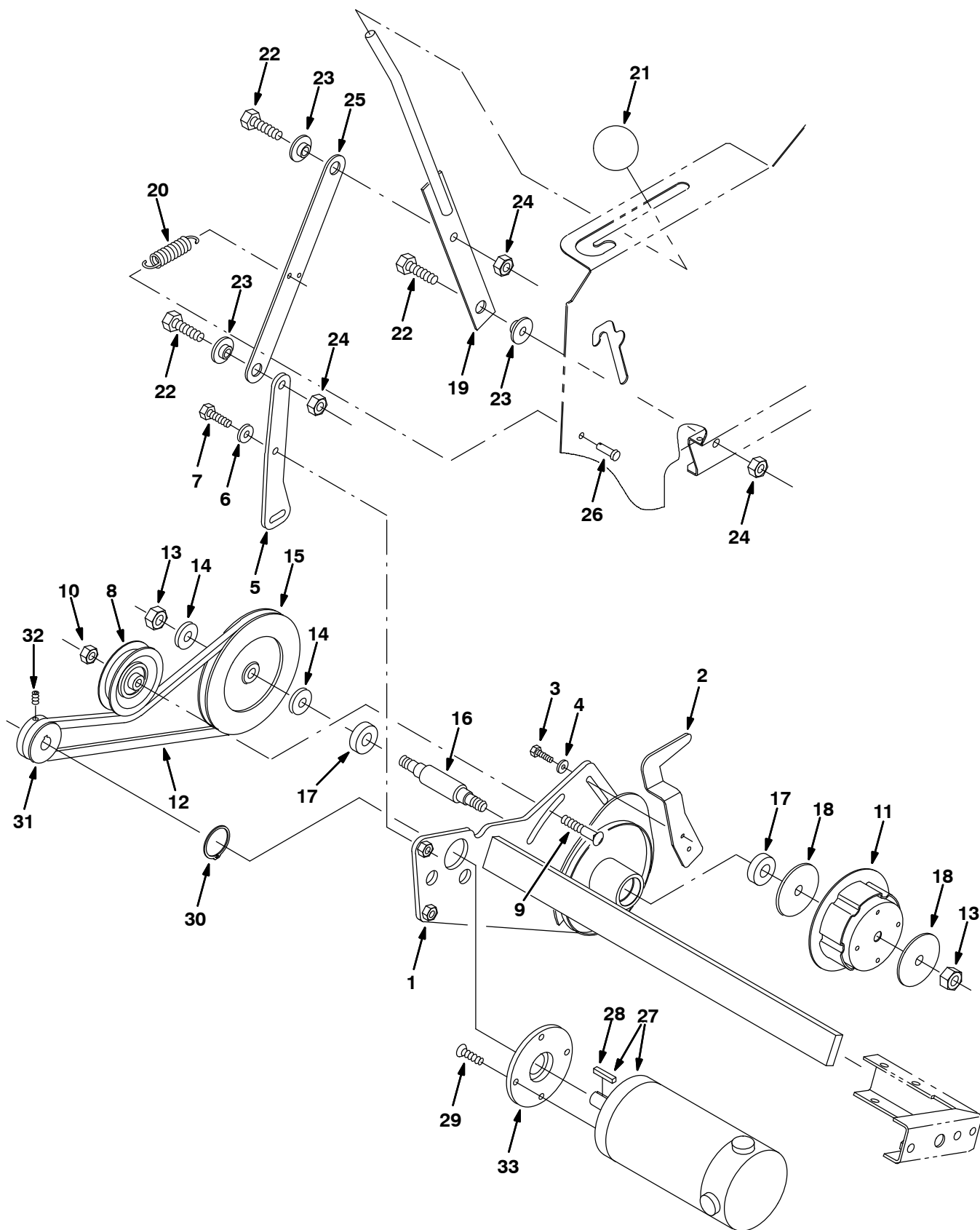
Fig. 22 – Main Brush Drive Group — Kehrwalzeantrieb-Gruppe — Groupe entraînement de la brosse principale
