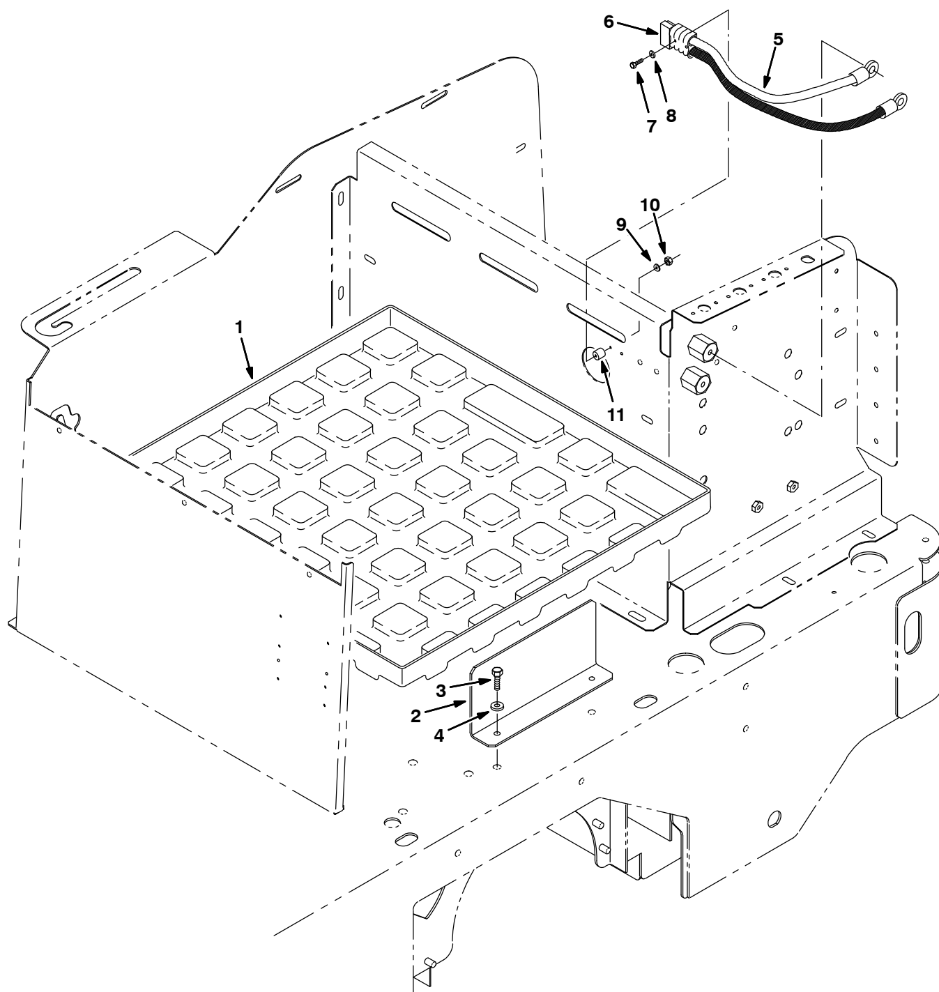
Fig. 29 – Battery Tray Group — Batterie Träger Gruppe — Groupe Batterie Porteur
