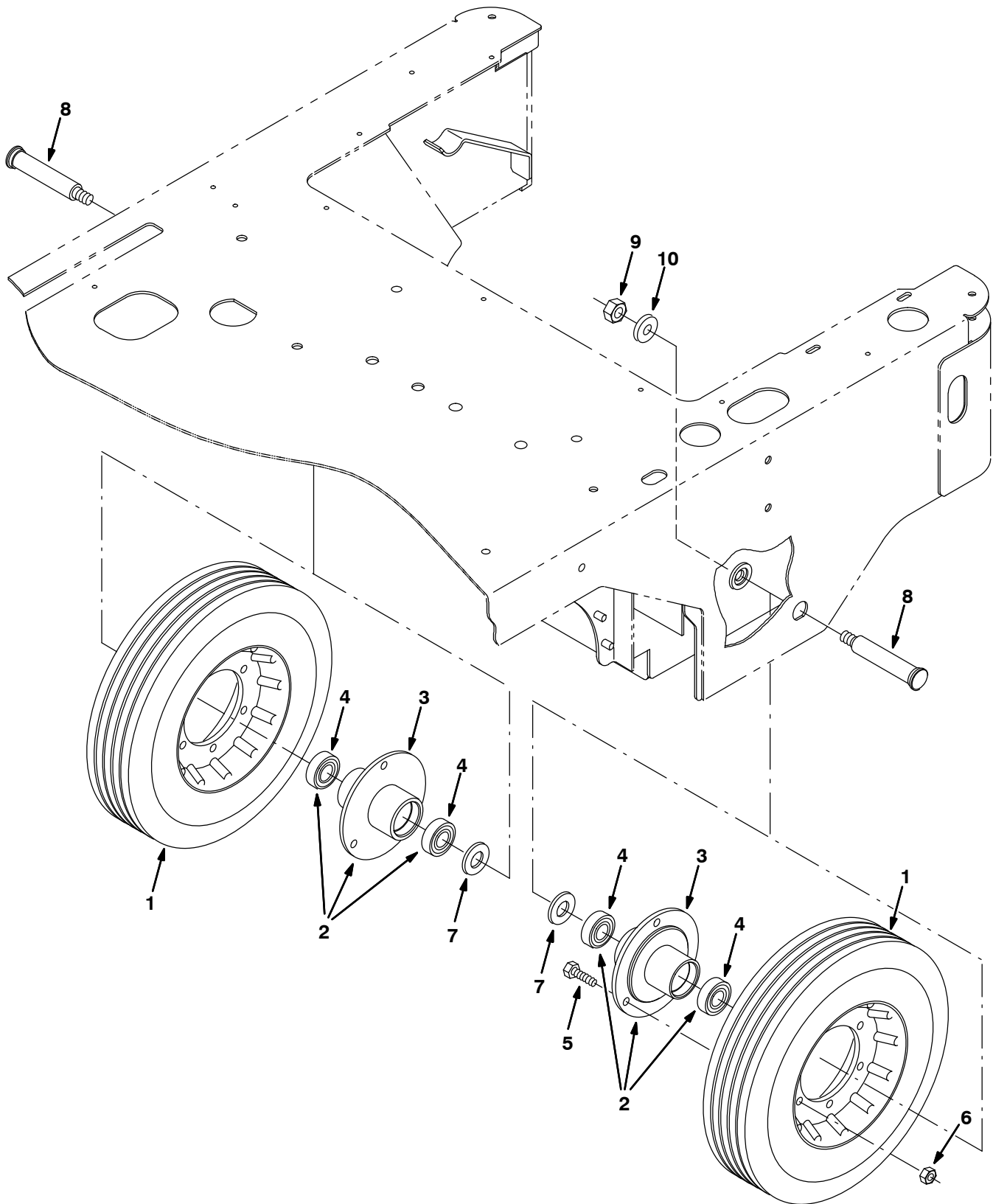
Fig. 17 – Rear Wheel Group — Heckrad-Gruppe — Groupe roue arrière
