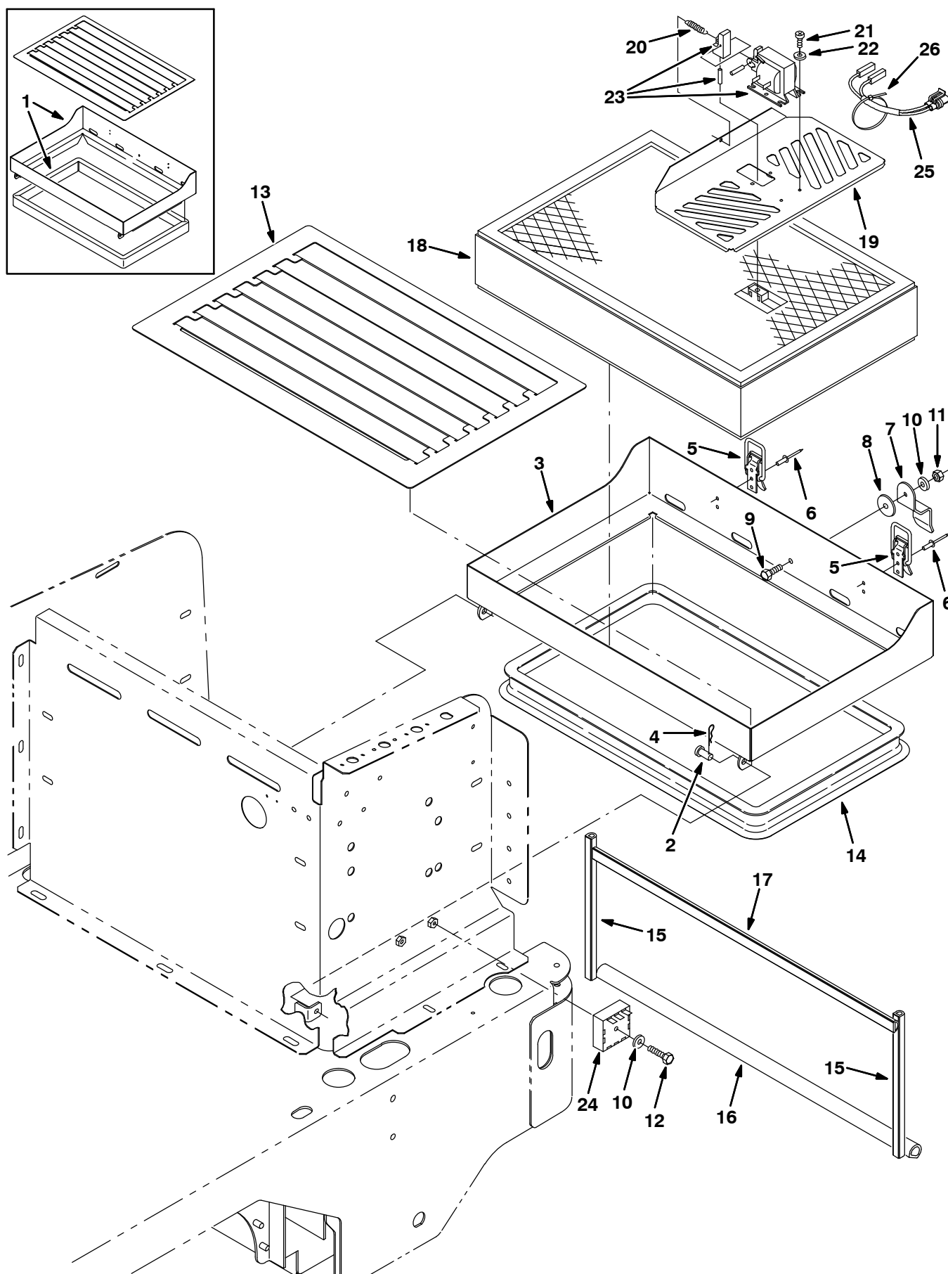
Fig. 28 – Filter Shaker Group — Filter-Rüttler-Gruppe — Groupe secoueur du filtre
