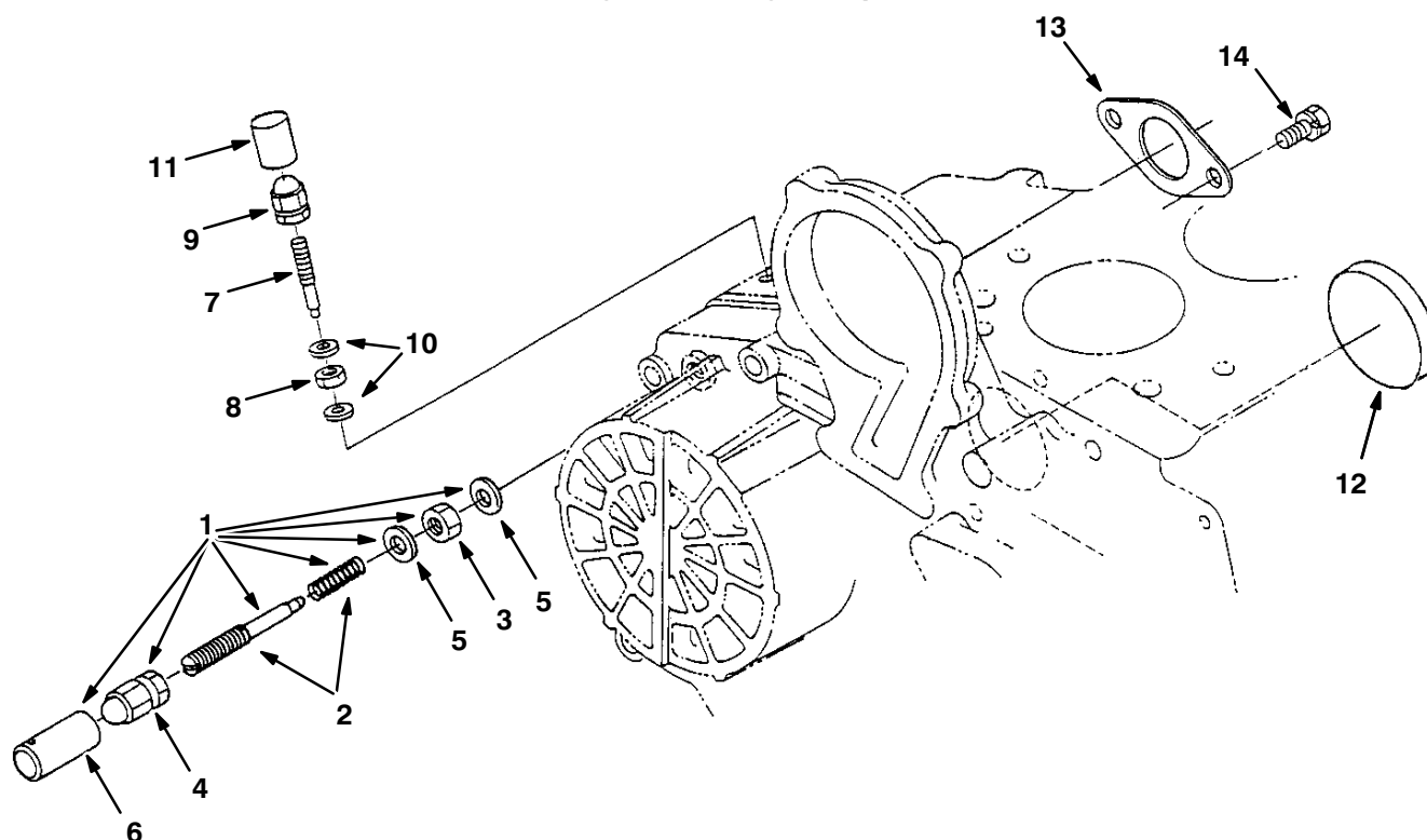
Fig. 18 – Idling Group
