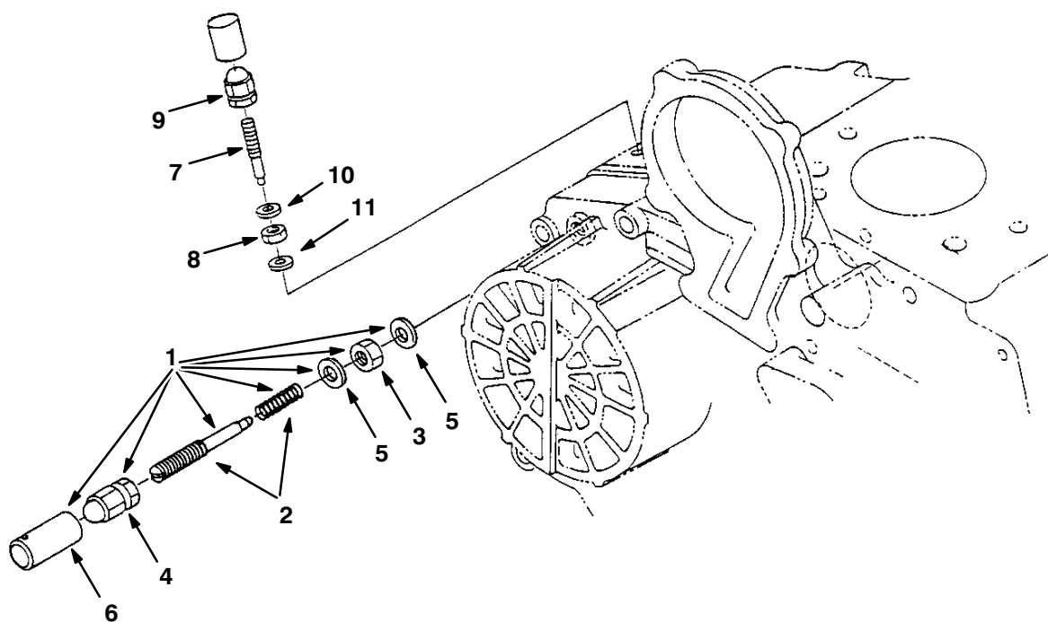
Fig. 19 – Idling Group
