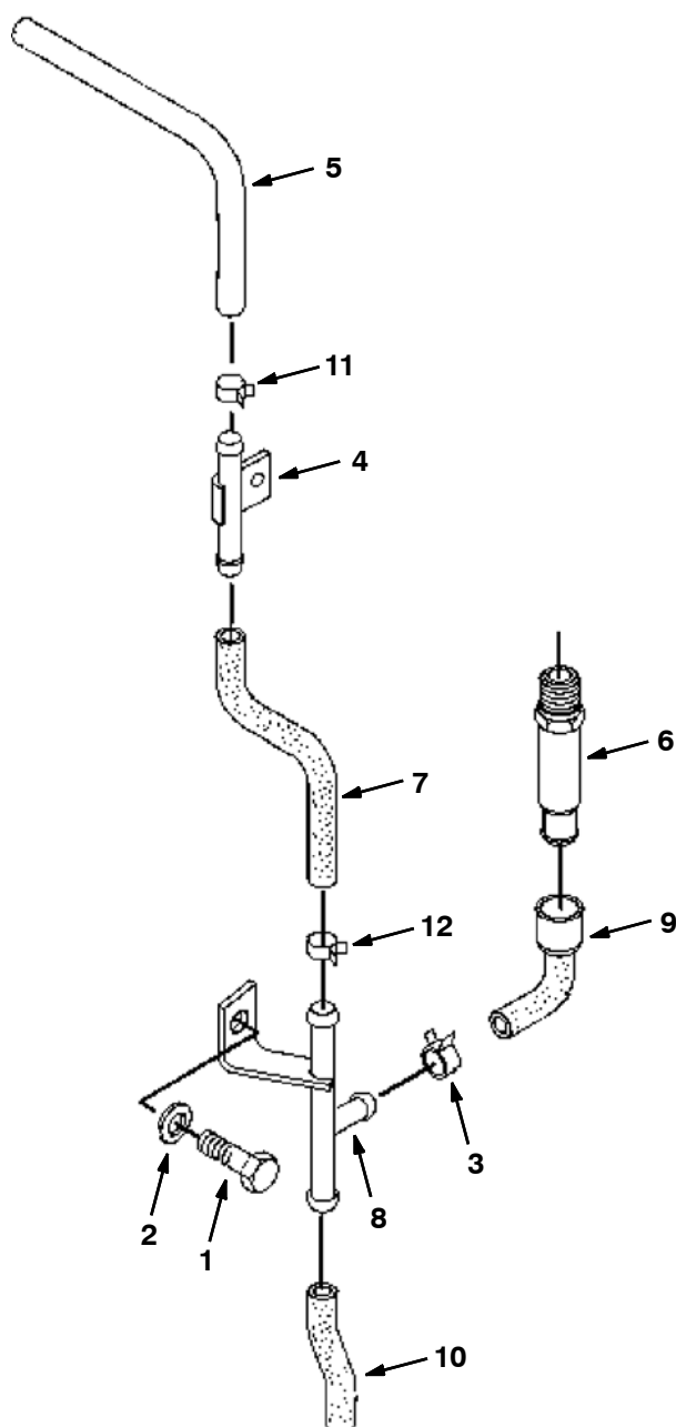
Fig. 14 - Fumes Disposal Group — Entlüfter-Gruppe — Groupe reniflard
