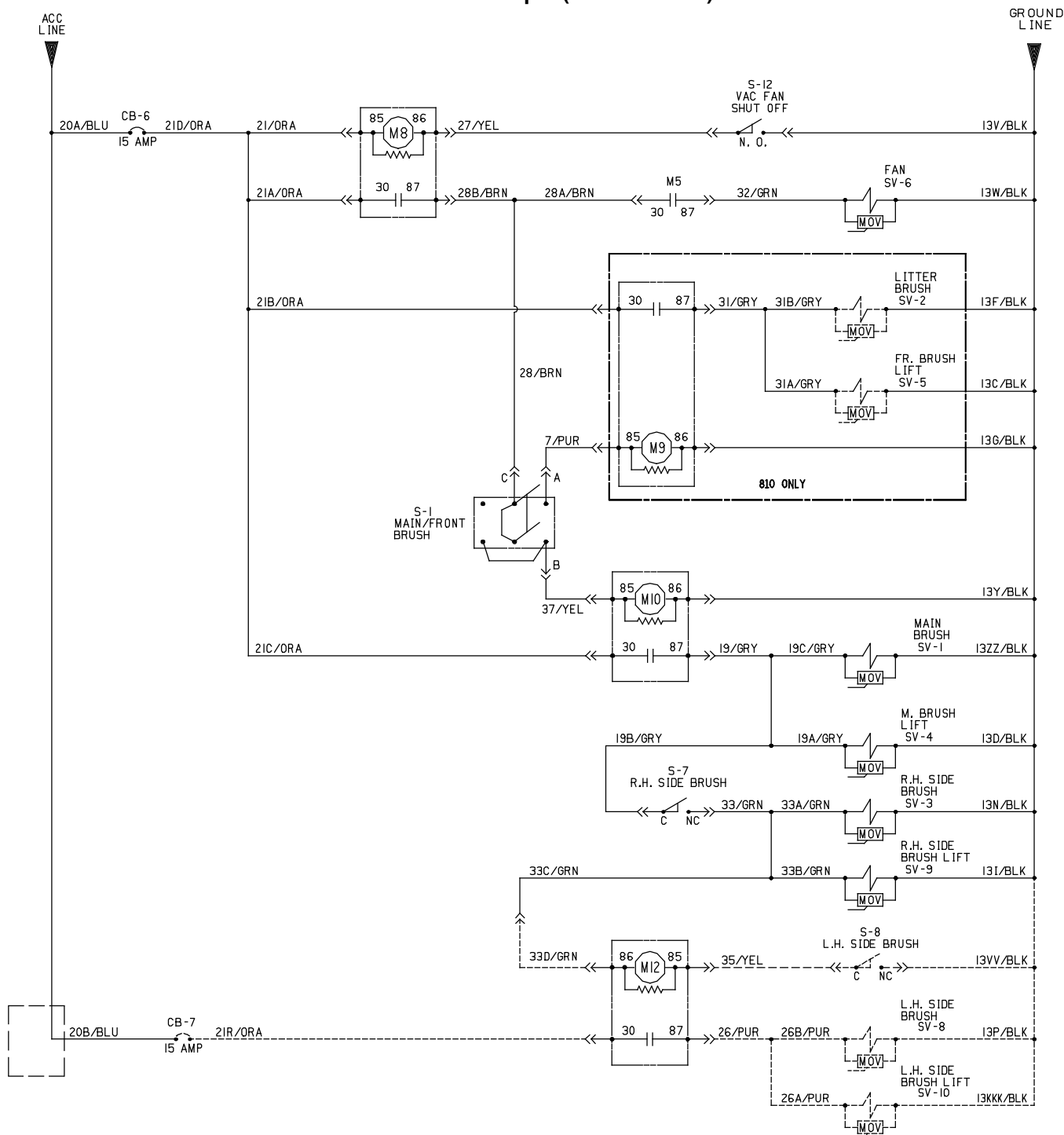
Fig. 61 - Electrical Schematic (006009- ) Elektroschaltbild (006009- ) Schéma Électrique (006009- )
