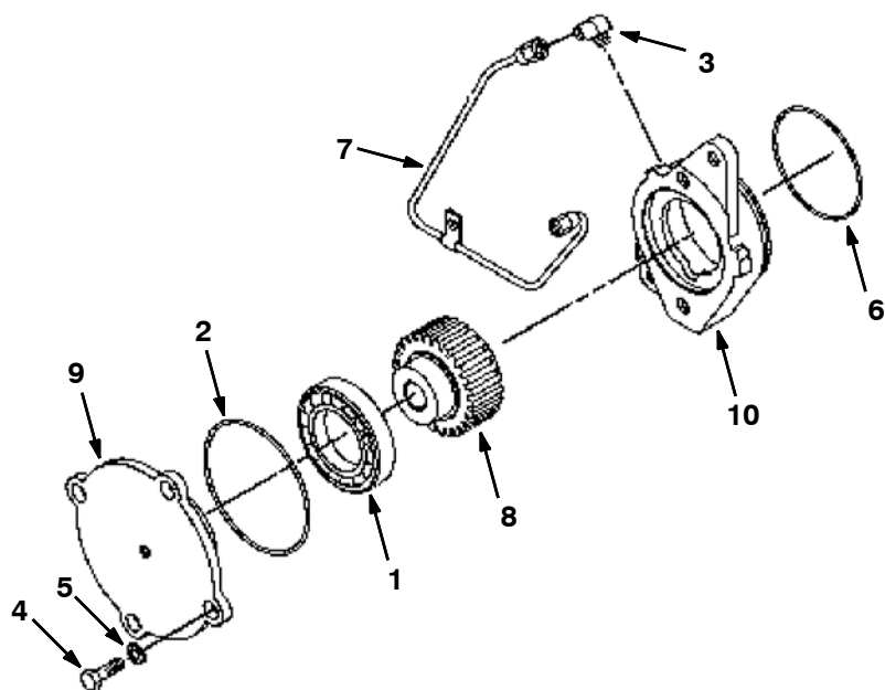
Fig. 8 - Auxiliary Drive Group — Nebenantriebseinheit — Groupe commande auxiliaire
