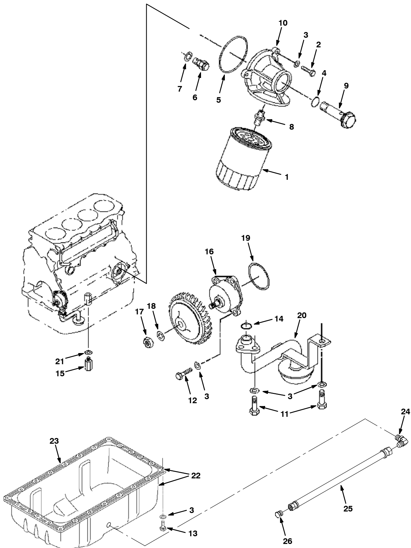
Fig. 9 - Oil Pan Group — Ölwannen-Gruppe — Groupe carter inférieur
