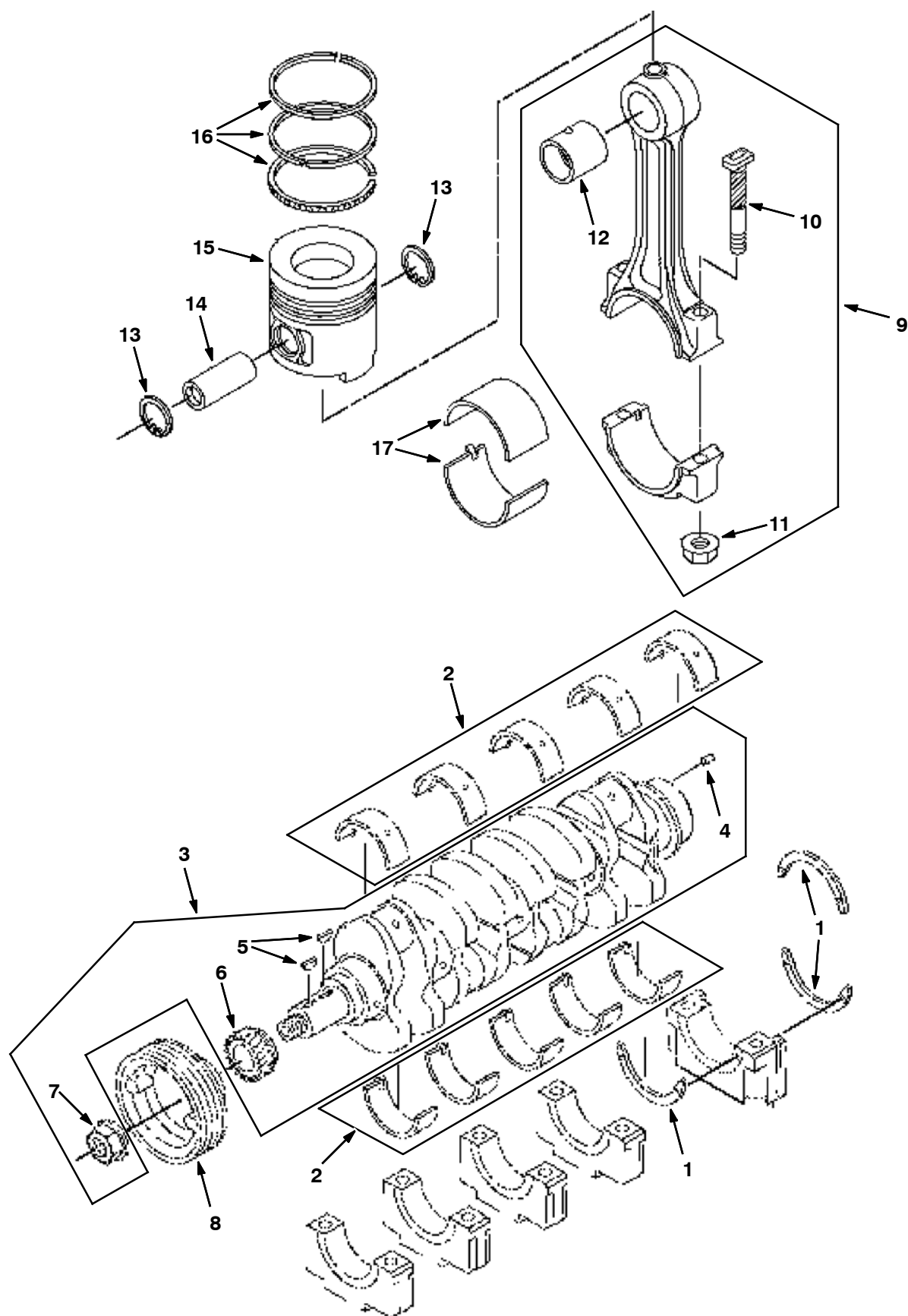
Fig. 2 - Crankshaft Group — Kurbelwellen-Gruppe — Groupe carter de vilebrequin
