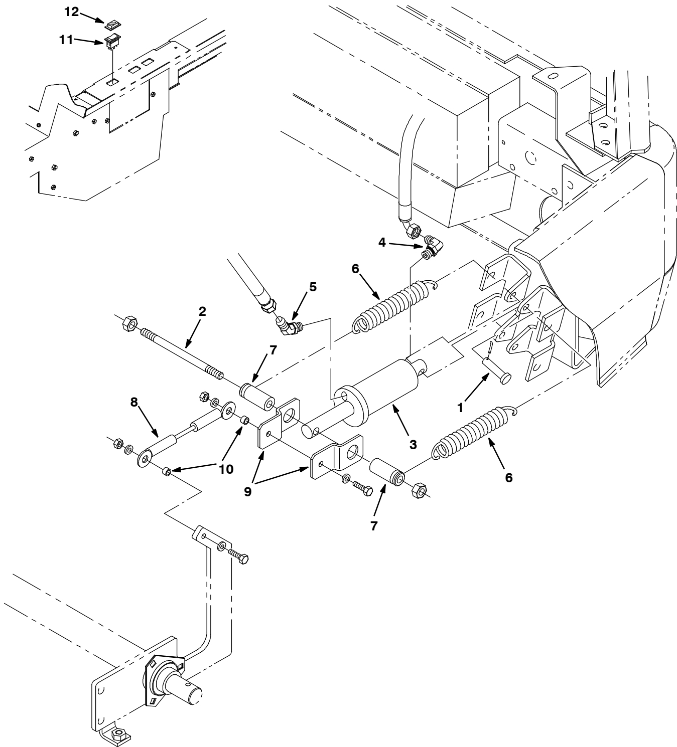
Fig. 52 - Main Brush Lift Group Kehrwalzehub-Gruppe Groupe levage de la brosse principale
