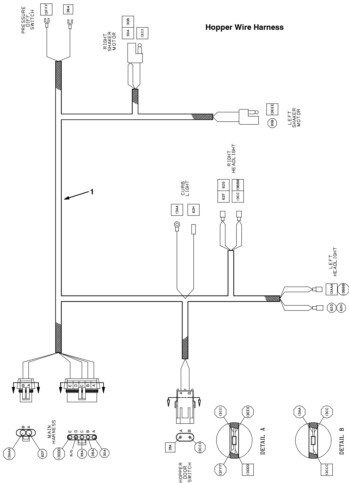
Fig. 63 - Wire Harnesses Group, Diesel, Hopper (004000- ) Kabelstrang-Gruppe (004000- ) Groupe faisceau de fils (004000- )
