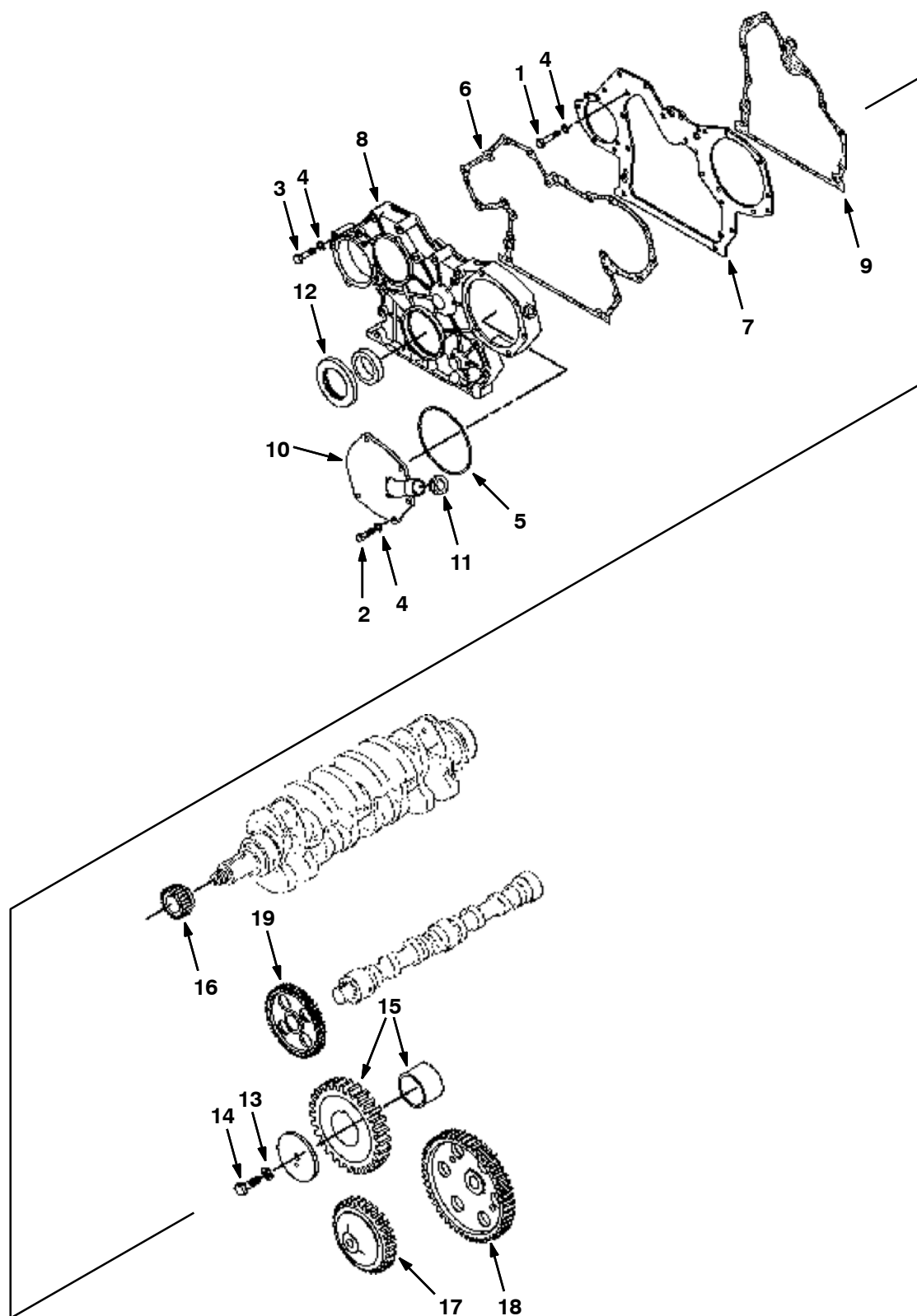
Fig. 6 - Front Cover Group — Vorderhauben-Gruppe — Groupe couvercle avant
