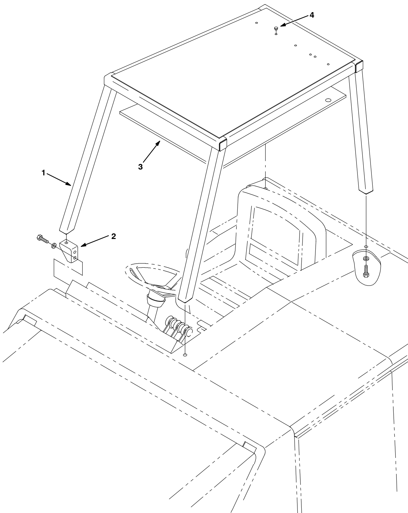
Fig. 9 - Overhead Guard Kit — Überkopf-Schutz-Satz — Jeu de pièces protège-conducteur
