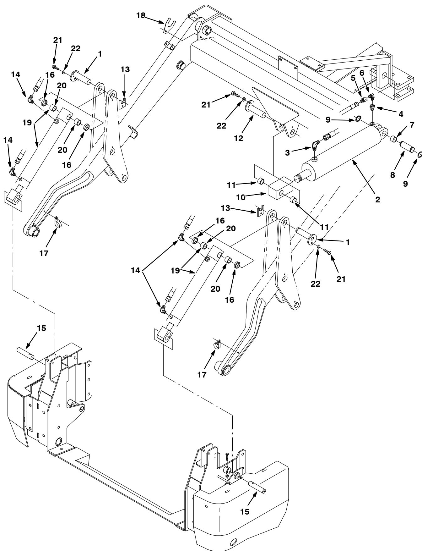
Fig. 12 - Hopper Cylinder Group Kehrichtbehälter-Zylinder-Gruppe Groupe cylindre trémie
