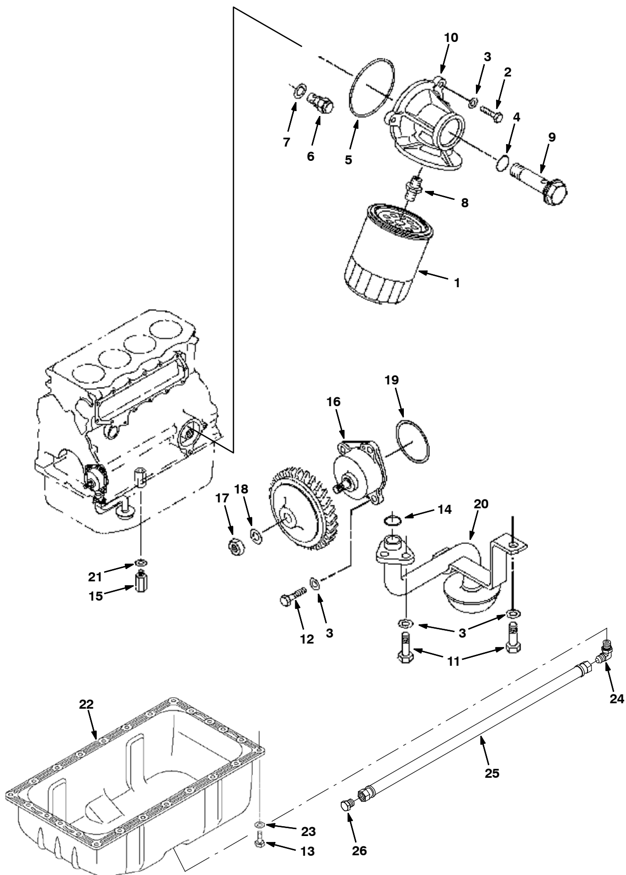
Fig. 9 - Oil Pan Group — Ölwannen-Gruppe — Groupe carter inférieur
