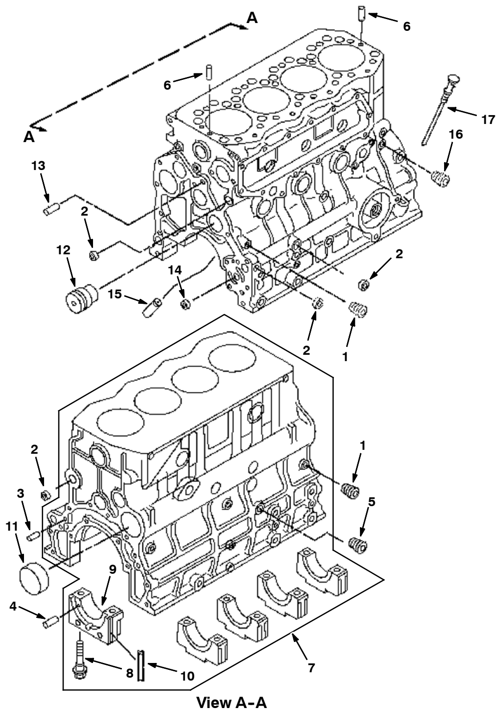
Fig. 1 - Cylinder Block Group — Zylinderblock-Gruppe — Groupe bloc cylindres
