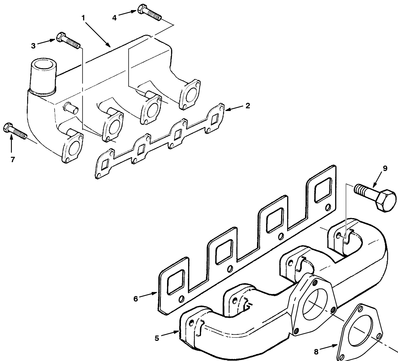
Fig. 16 - Manifold Group — Krümmergruppe — Groupe collecteur
