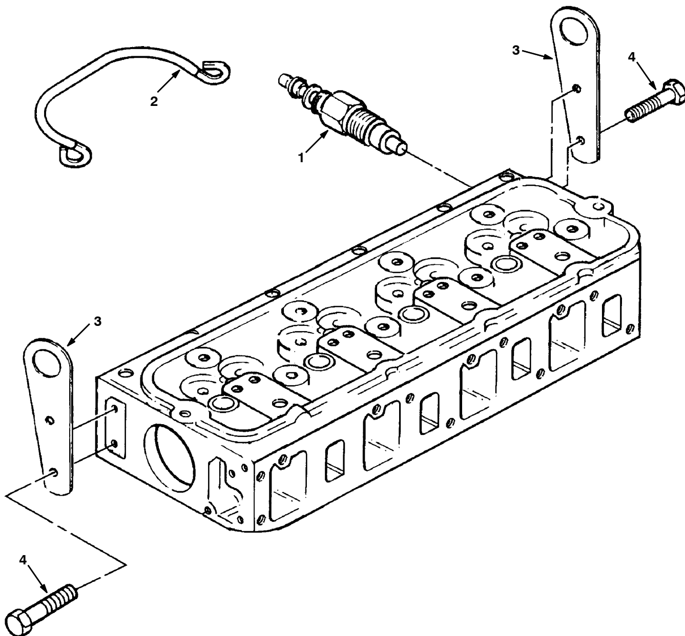
Fig. 17 - Glow Plug and Engine Lift Group — Glühkerzen- und Motoranhebe-Einheit — Groupe bougie de préchauffage et hauteur de gauchissage du moteur
