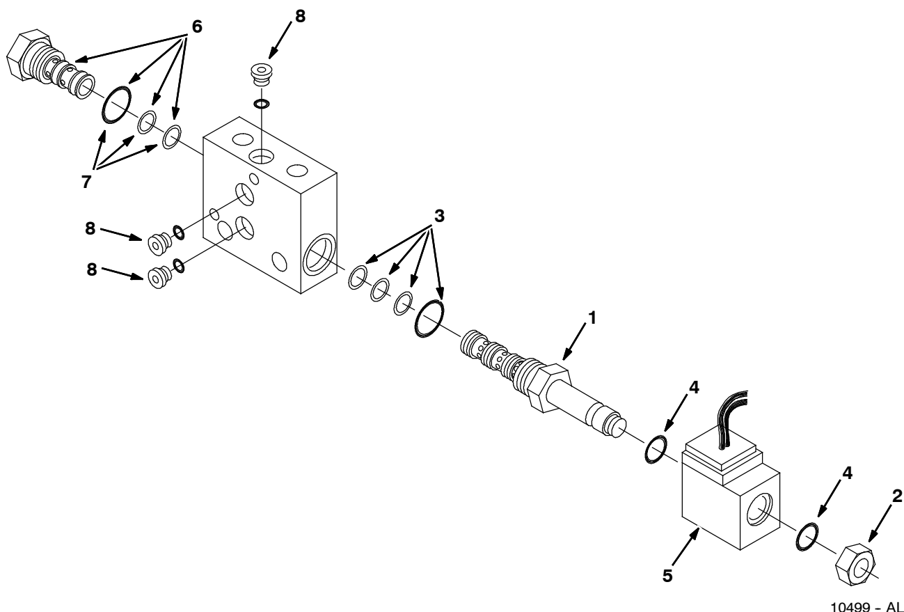
Fig. 24 - Hydraulic Solenoid Valve Breakdown, 84016 — Hydraulik-Zugmagnetventil-Komponente — Composantes soupape magnétique du système hydraulique
