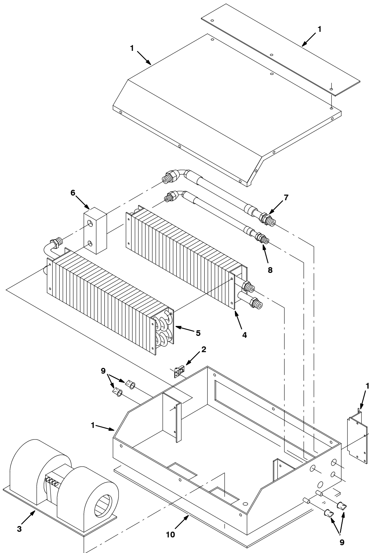
Fig. 32 - AC and Heater Box Breakdown, 380613 — Komponente des Luftkonditionierungs- und Heizungsgehäuses — Elément de boîtier de climatisation et radiateur
