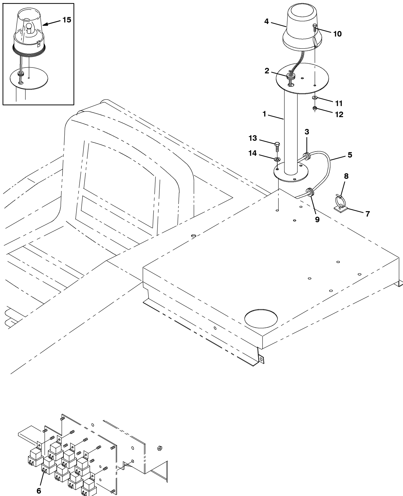
Fig. 6 - Revolving Light Kit, Low — Blinklicht-Satz, LRC — Jeu de pièces gyrophare, côtés droit et gauche
