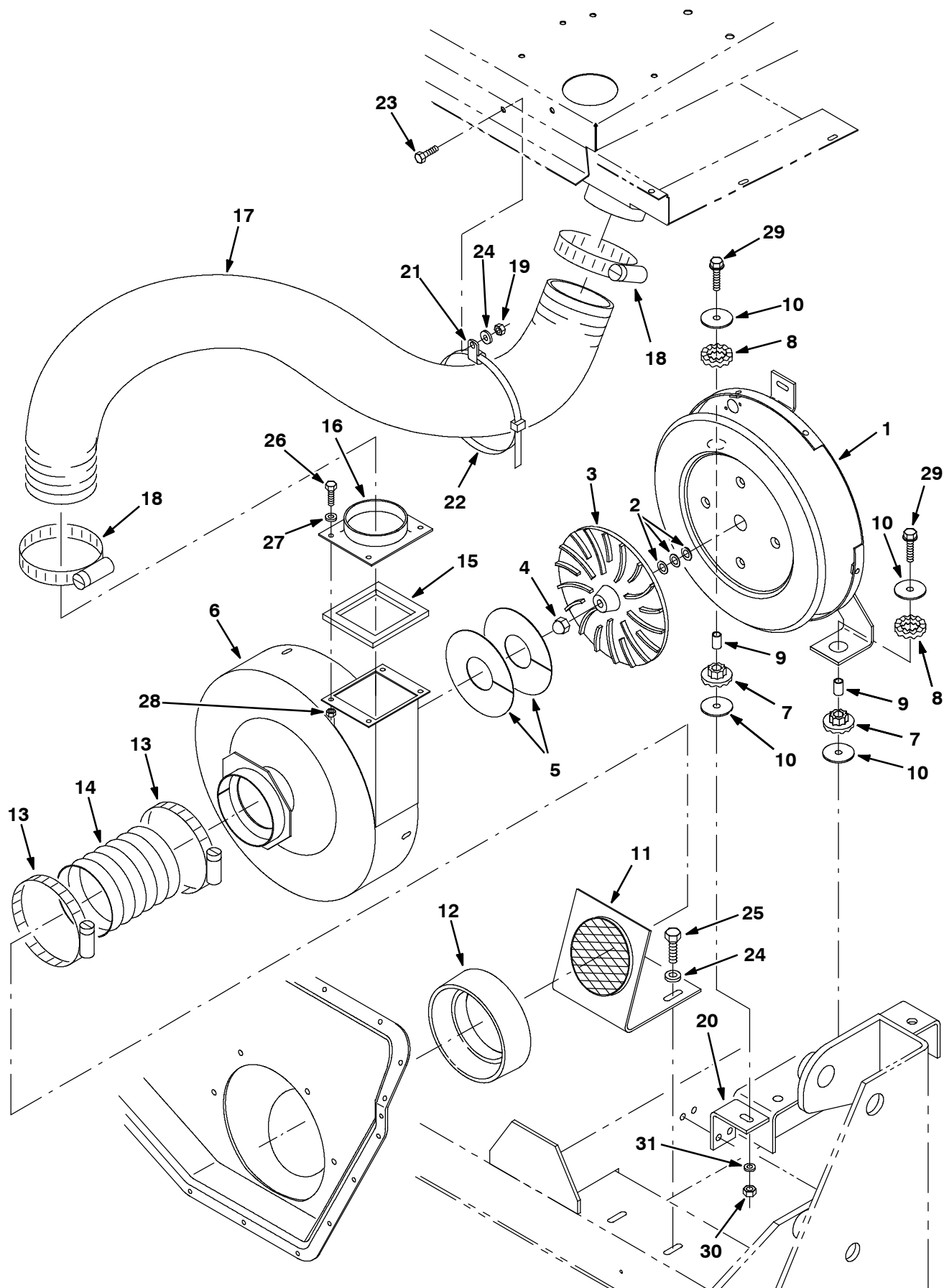
Fig. 54 - Vacuum Fan Group Vakuumgebläse-Gruppe Groupe extracteur
