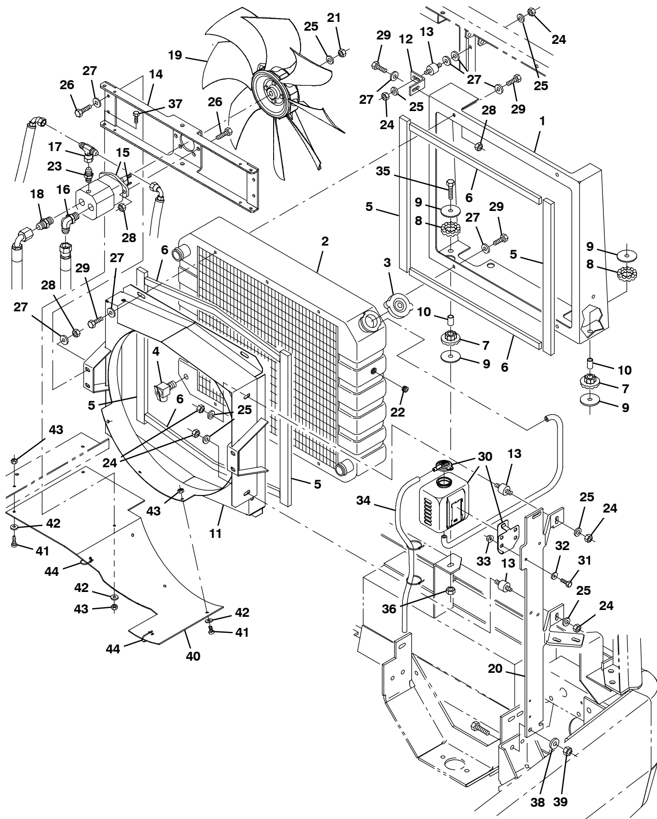
Fig. 34 - Radiator Group (007000- ) Kühlergruppe (007000- ) Groupe radiateur (007000- )
