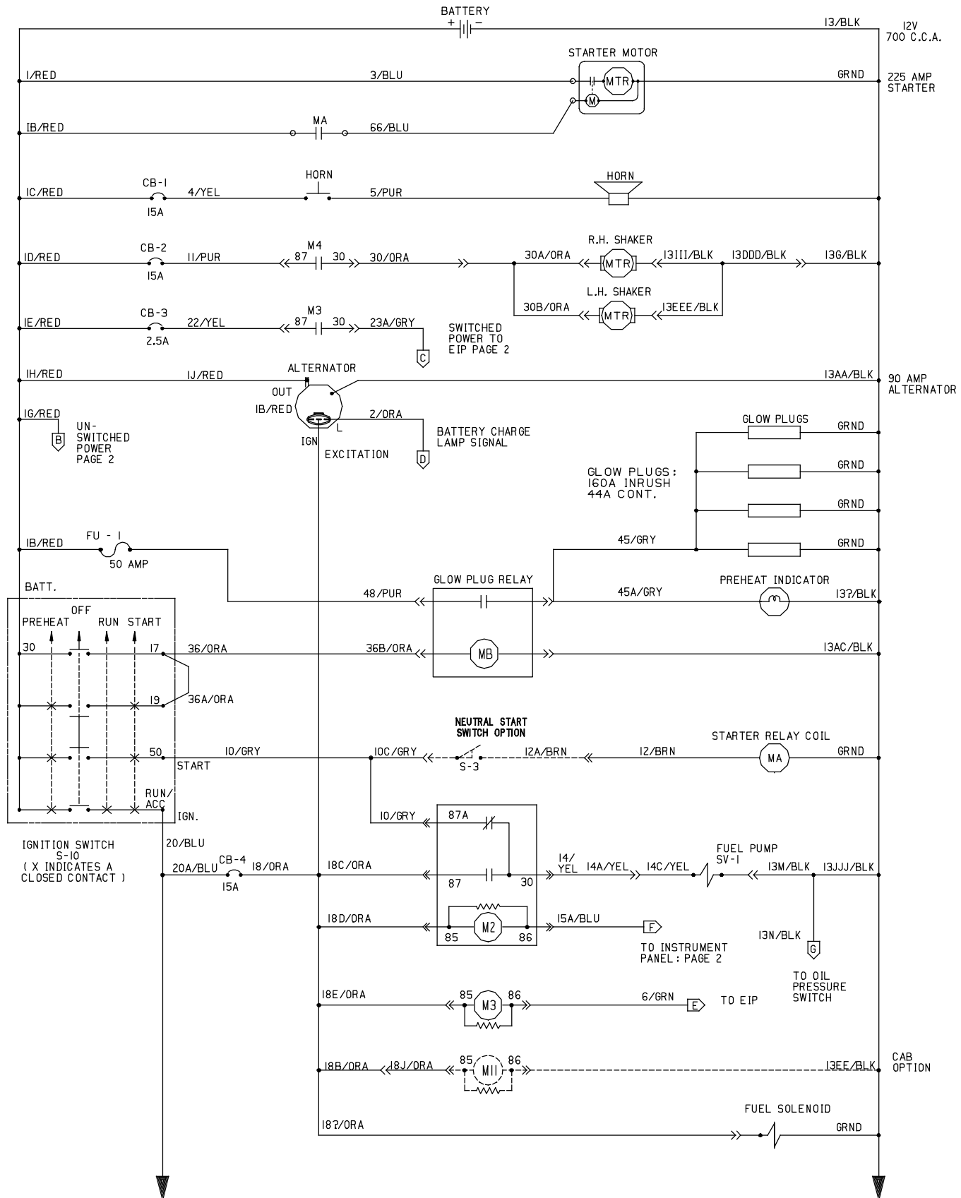
Fig. 61 - Electrical Schematic (006009- ) Elektroschaltbild (006009- ) Schéma Électrique (006009- )
