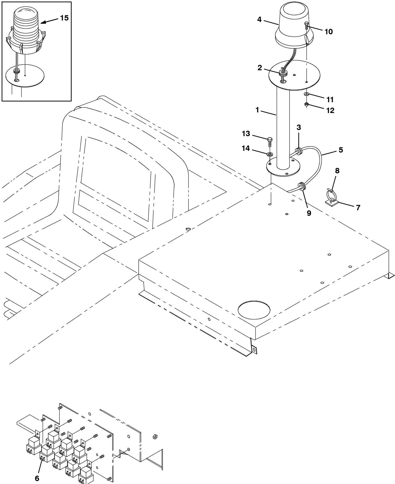
Fig. 5 - Flashing Light Kit, Low — Blinklicht-Satz LRC — Jeu de pièces gyrophare, côtés droit et gauche
