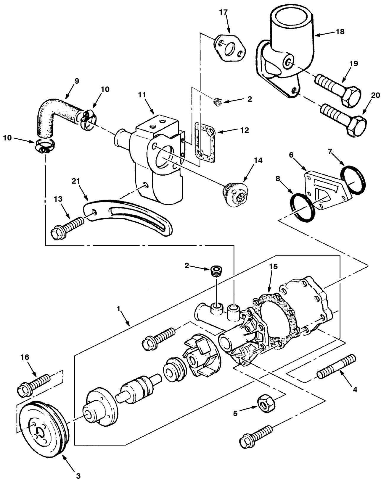
Fig. 15 - Water Pump Group — Wasserpumpen-Gruppe — Groupe pompe à eau
