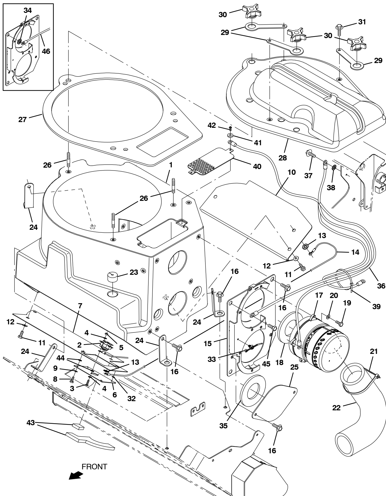
Fig. 38 – Hopper Vacuum Fan Group
