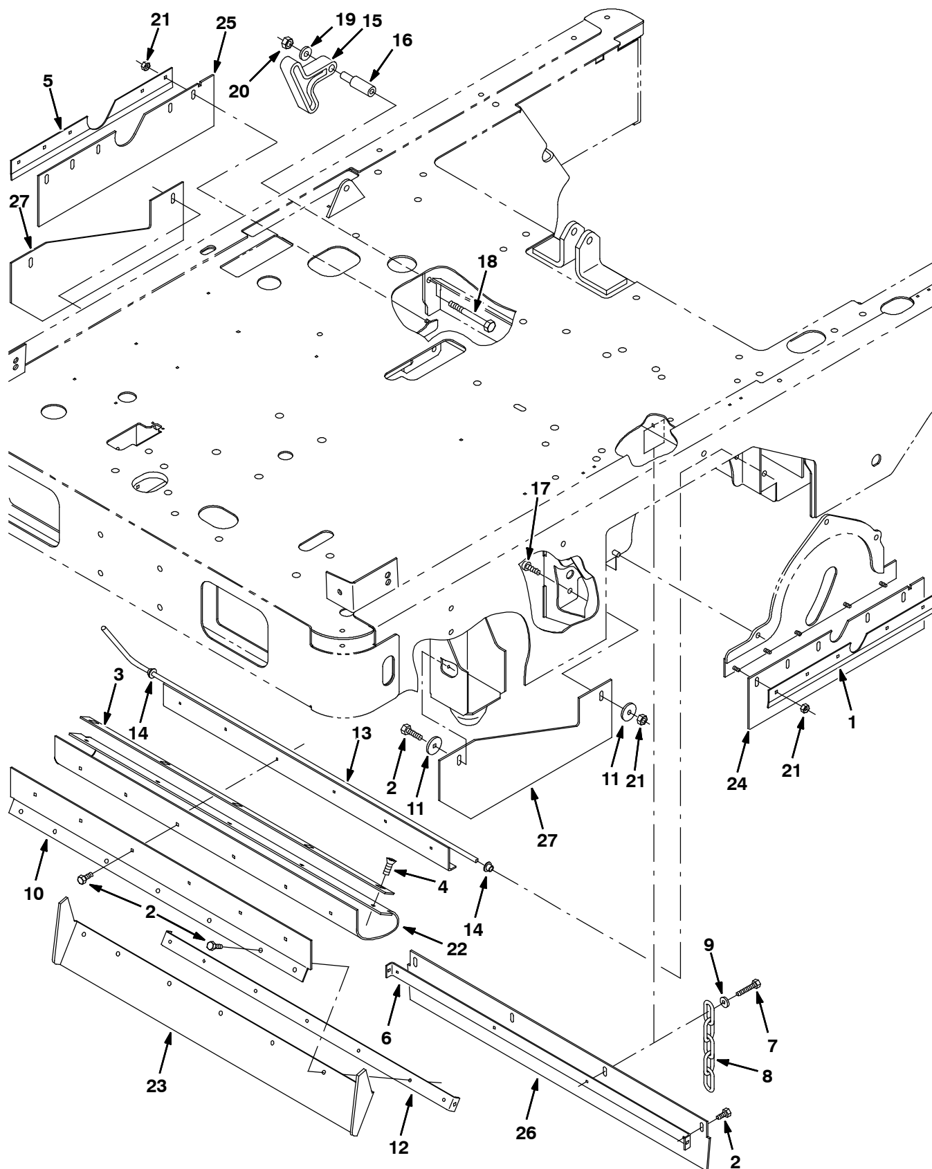
Fig. 16 - Main Brush Skirts Group — Hauptbürsten-Schürzen-Gruppe — Groupe jupes de la brosse principale
