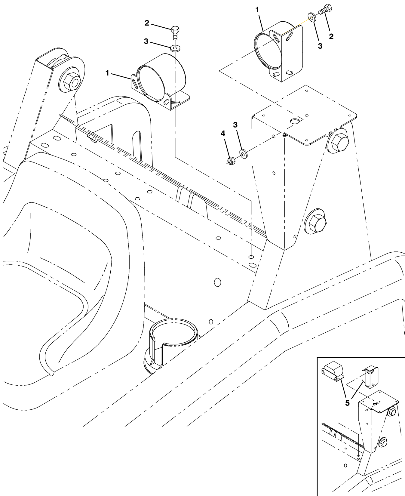
Fig. 16 - Backup Alarm Group — Rückfahr-Alarm-Gruppe — Groupe alarme de sécurité
