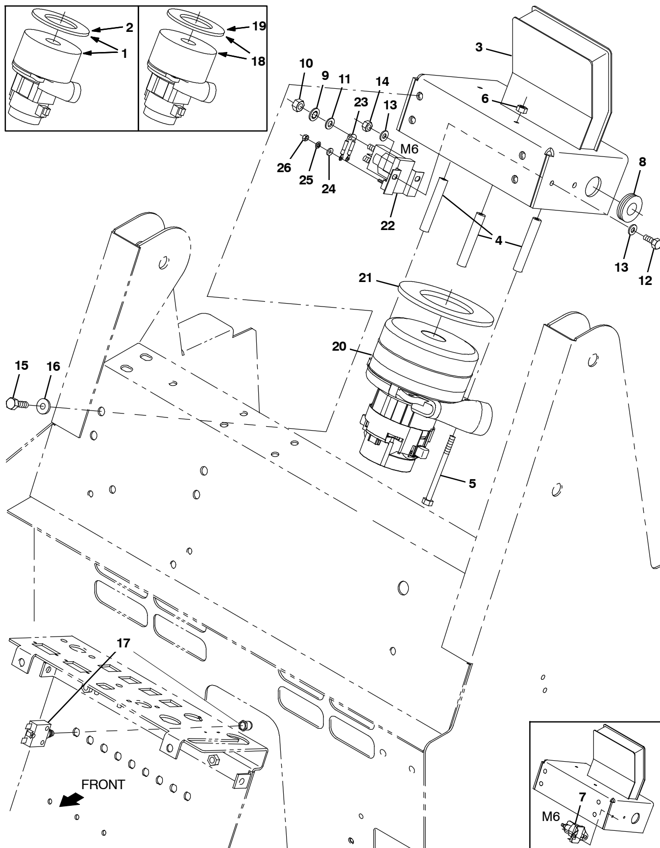
Fig. 4 - Vacuum Wand Fan Group — Saugstab-Ventilator-Gruppe — Groupe extracteur manche d'aspiration
