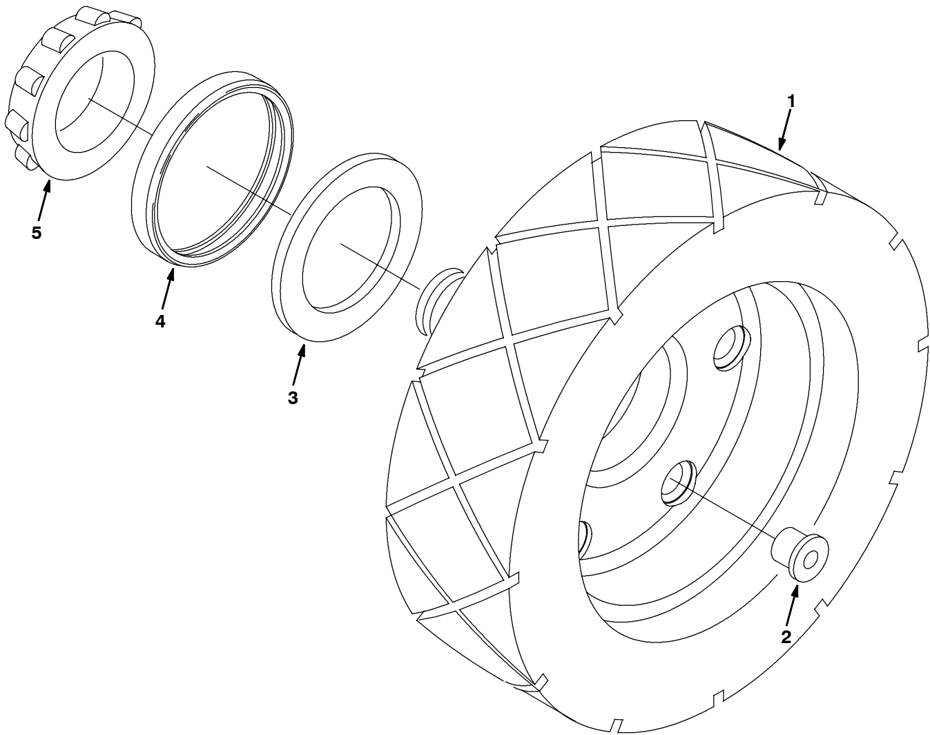
Fig. 27 - Solid Non-Marking Tire Assembly, Front — Vollgummi nicht markierender Reifen und Radsatz, Vorn — Ensemble bandage plein non marquant et roue, avant
