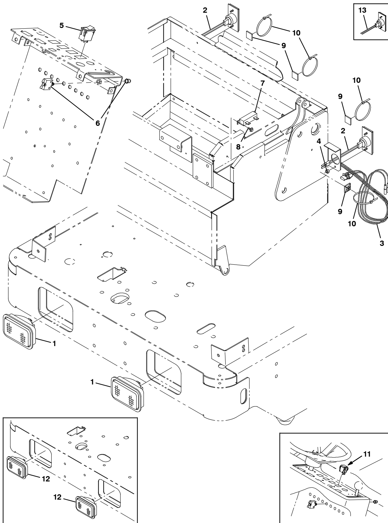
Fig. 15 - Light Kit — Licht-Satz — Jeu de pièces feu
