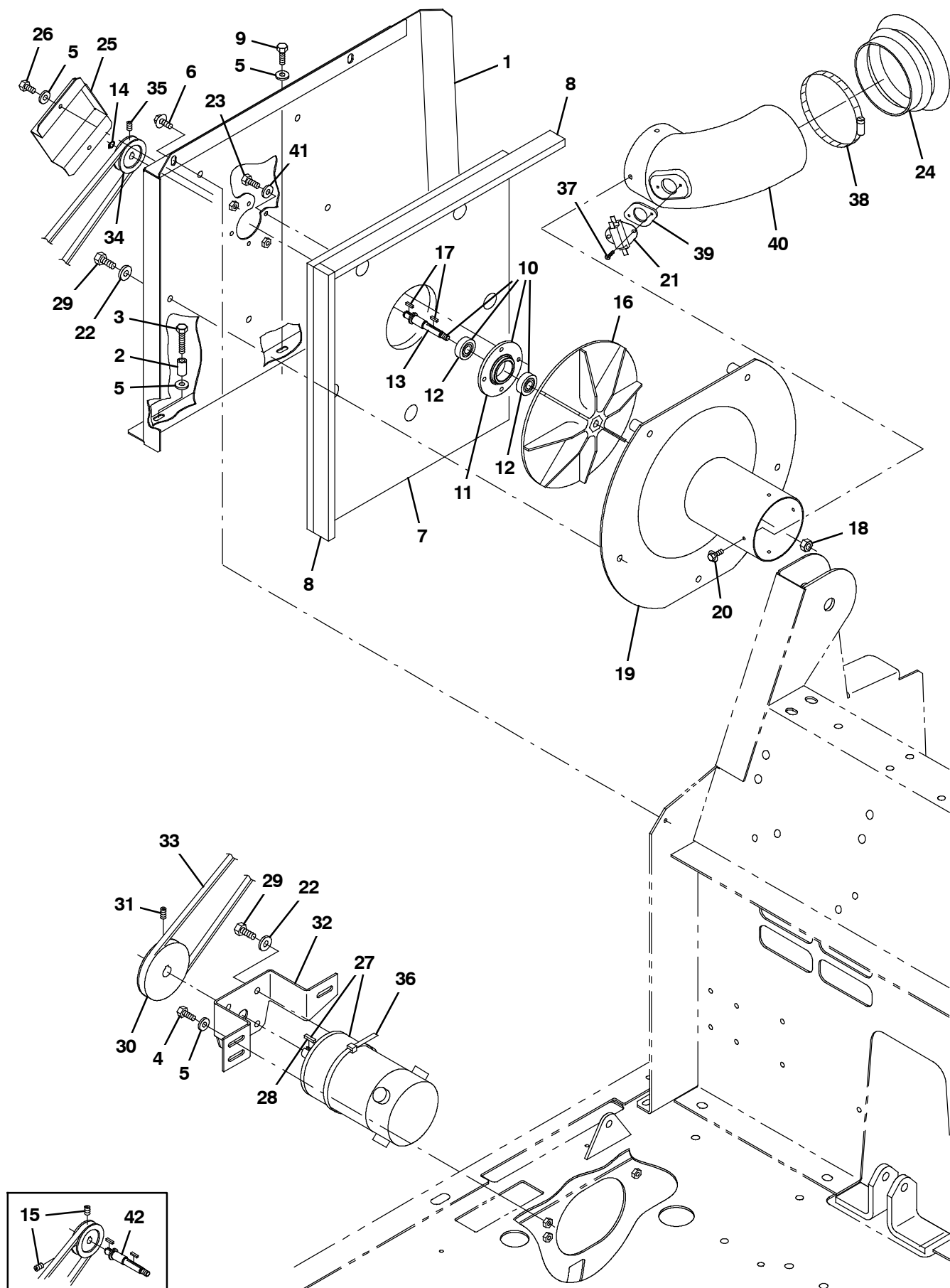
Fig. 22 - Vacuum Fan Group — Vakuümgebläse-Gruppe — Groupe extracteur
